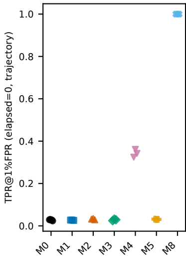
cifar100
