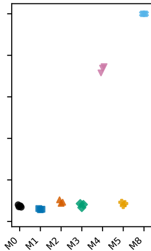
imagenet_r
