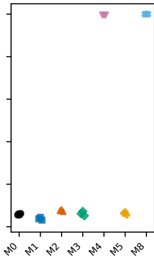
cub200
