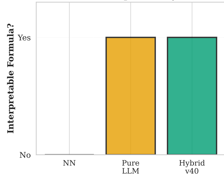
C: Interpretability
