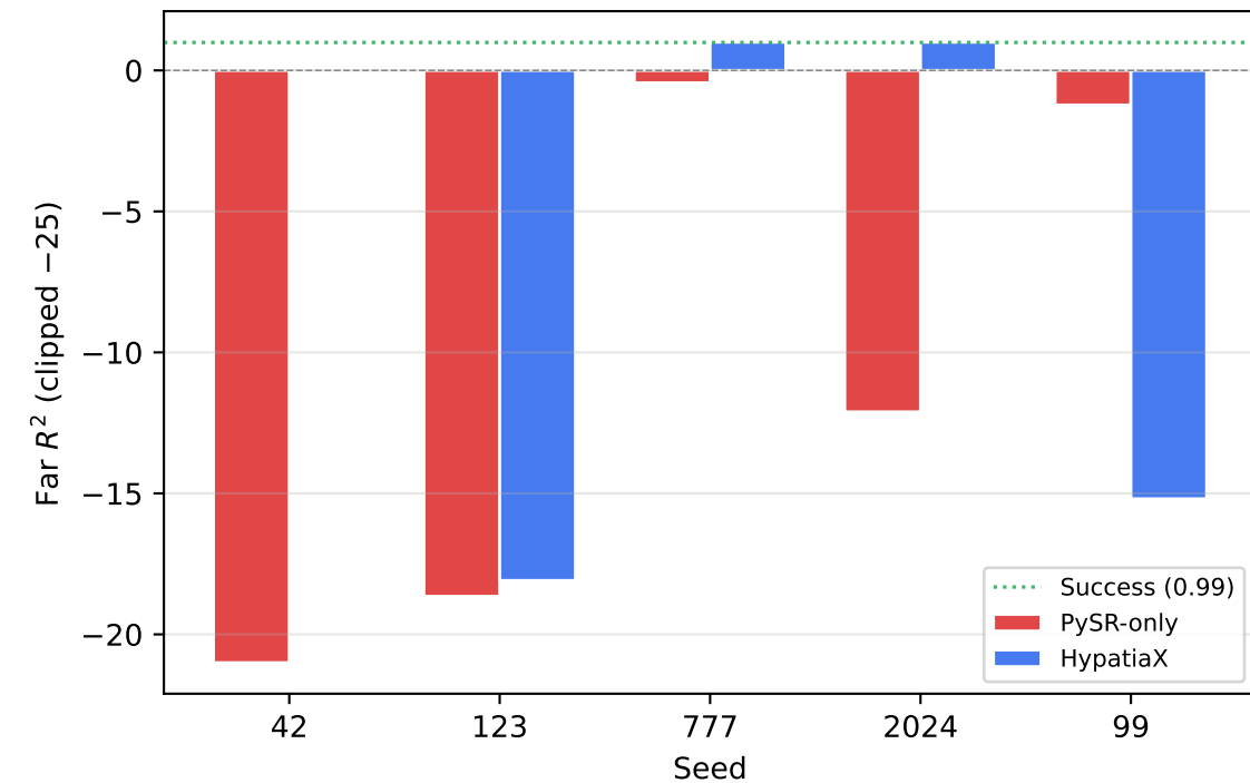
Far- R^2 per Seed
