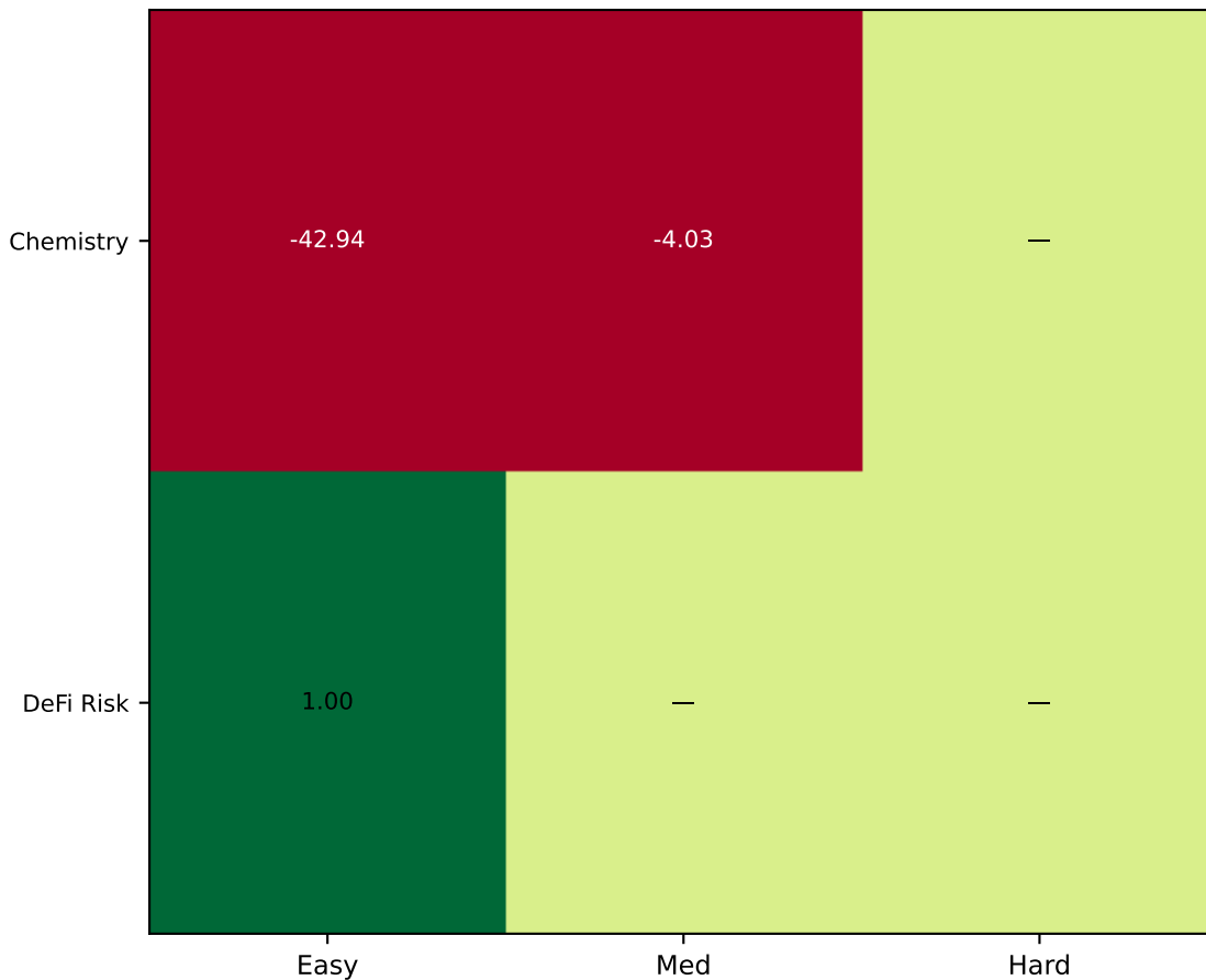
PySR-only
