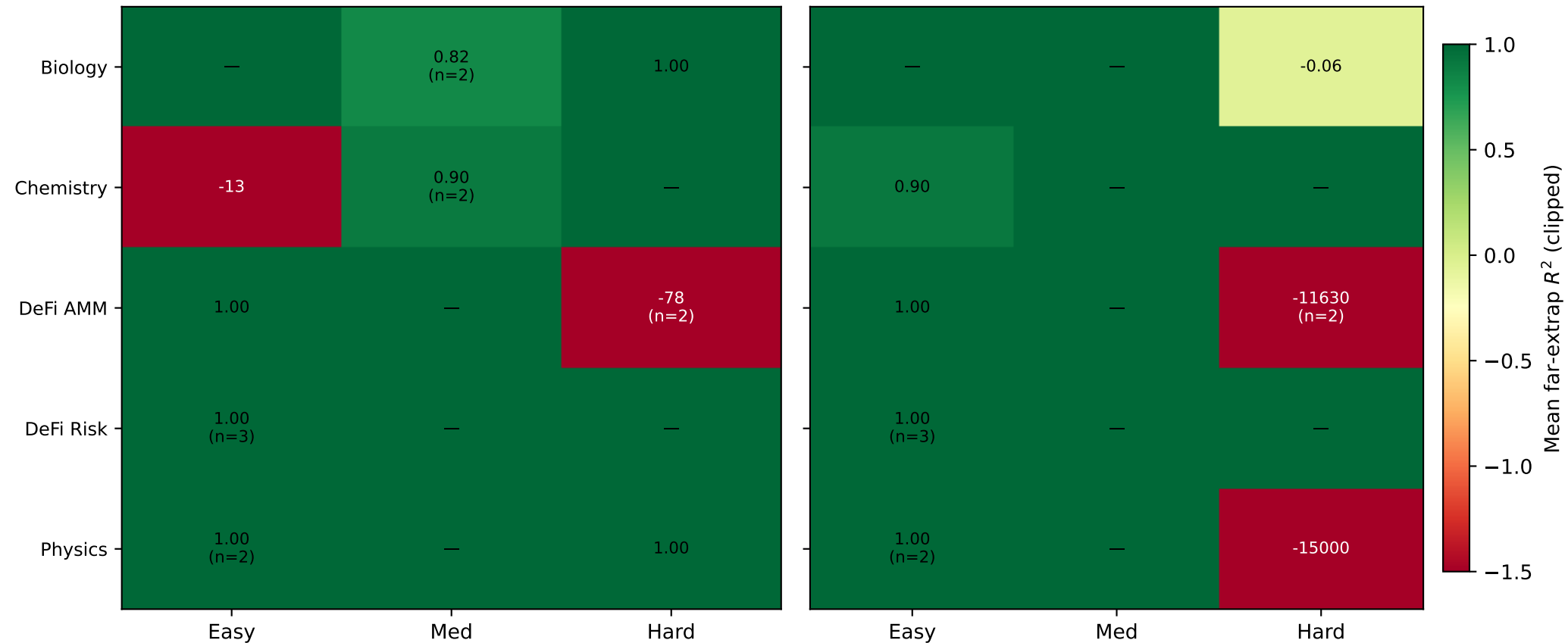
PySR-only
