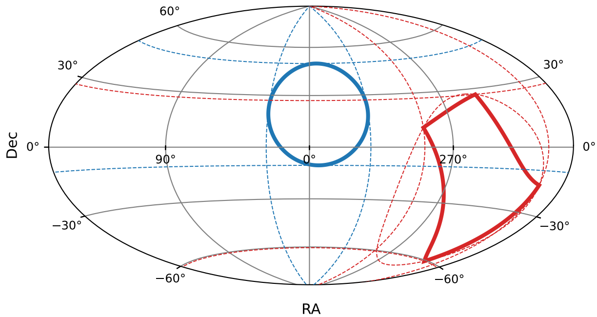
ICRS coordinates
