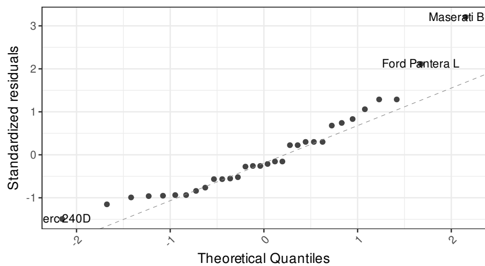
Normal Q-Q
