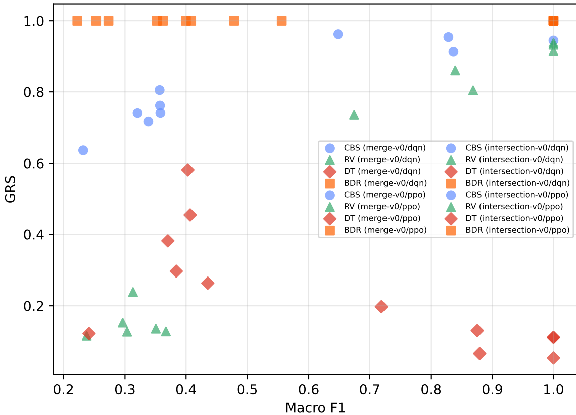
F1 vs GRS — Highway Environments
