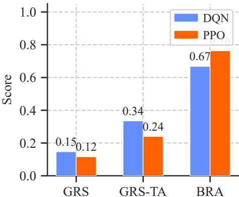
(a) CBS: PPO vs DQN
