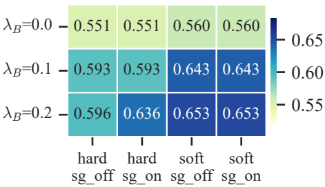
LunarLander -- Macro-F1
