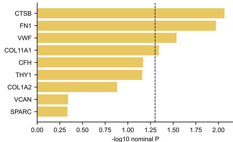
Protein context No candidate met FDR<0.05
