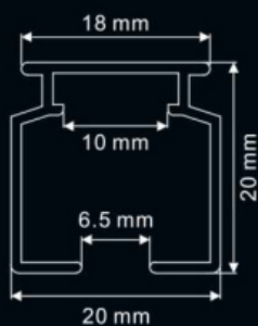
内轨
