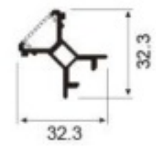
JNW-XT1010 inside 90° slim corner Weight : 0.38 kg/m
