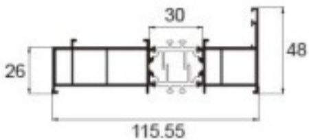
JNW-CT1711G 2.0 Outer Frame Weight : 1.93 kg/m
