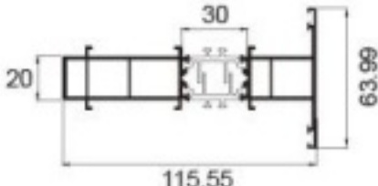
JNW-CT1713G 2.0 Center Column Weight : 2.06 kg/m
