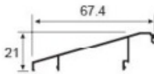
JNW-XT772 bevelled edge clip Weight : 0.32 kg/m
