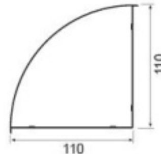
ZJ110A 110 corner-90° Weight : 1.42 kg/m
