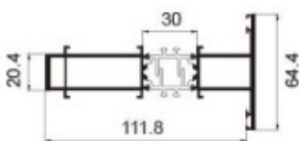
JNW-ZH783F 3.0 Center Column Weight : 2.27 kg/m
