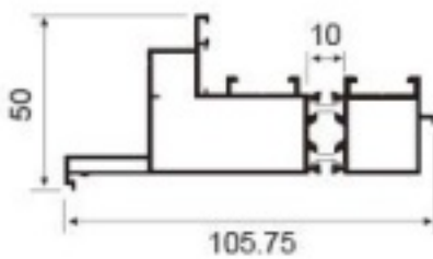
DZ-CT797F slim subframe Weight : 1.55 kg/m
