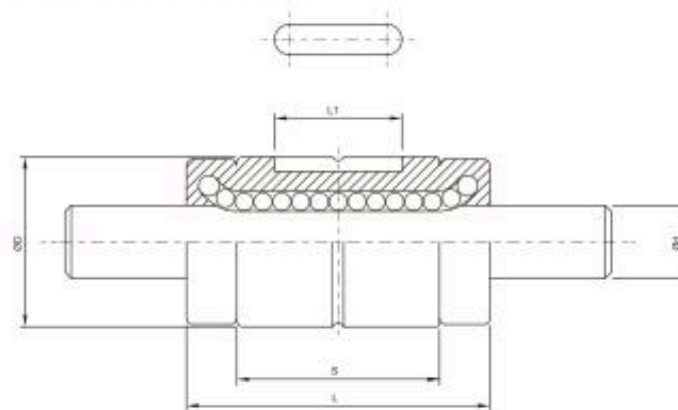
FSLT 系列规格尺寸表 FSLT Series Specification and Size Table
