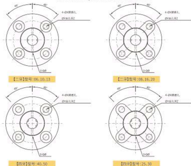
FSLF 系列规格尺寸表 FSLF Series Specification and Size Table
