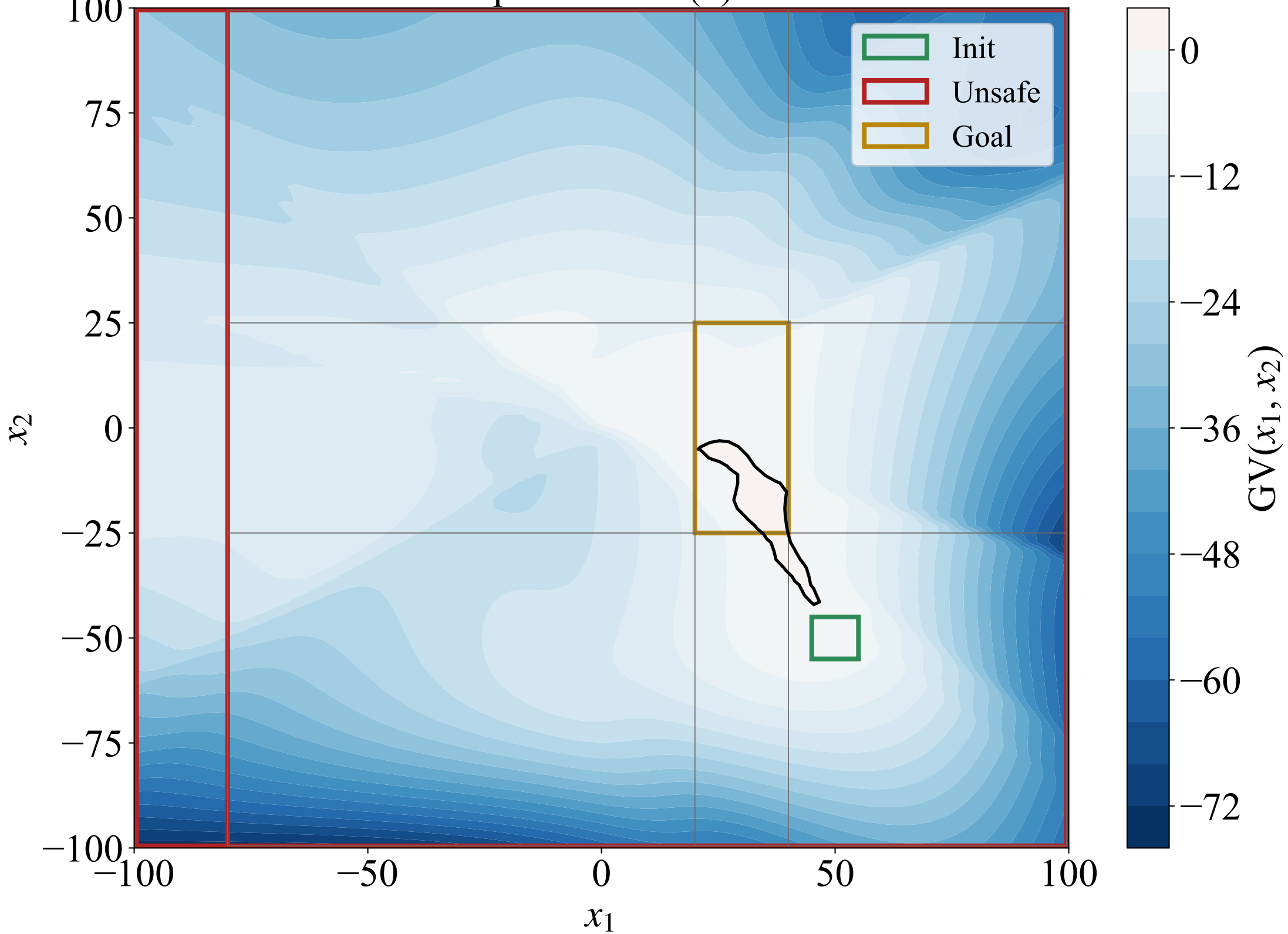
Epoch 0 - GV(x)
