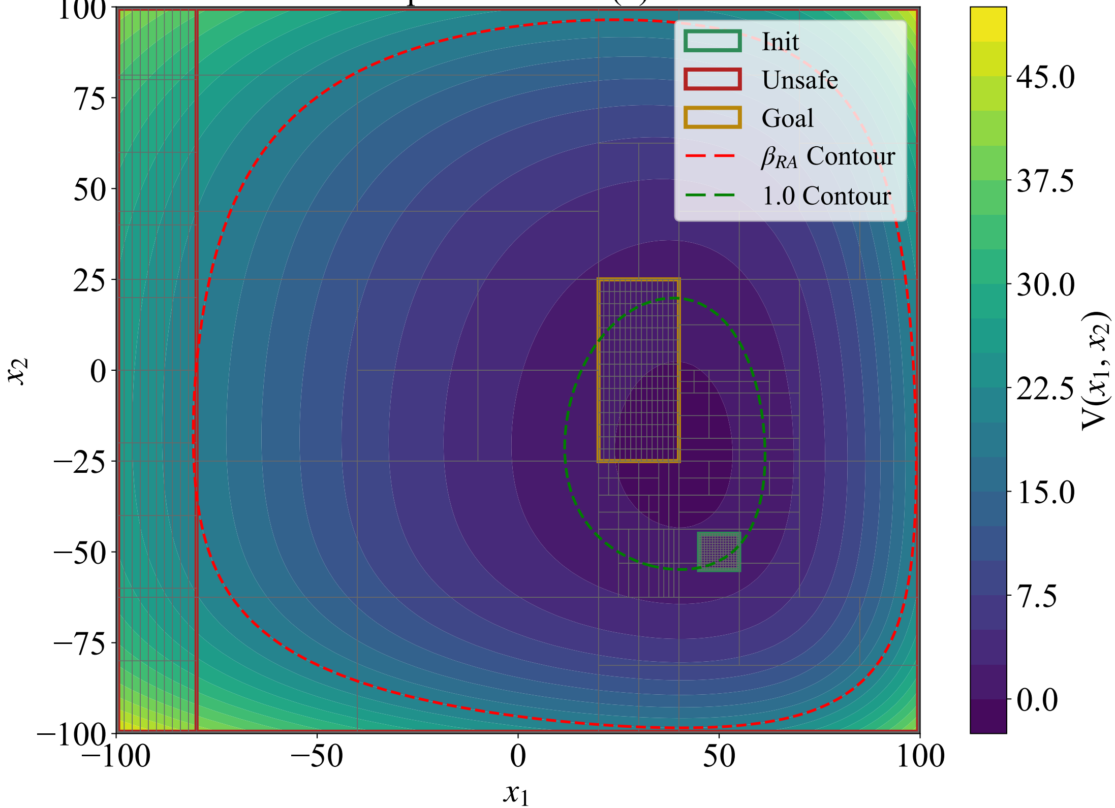
Epoch: 1000 - V(x)
