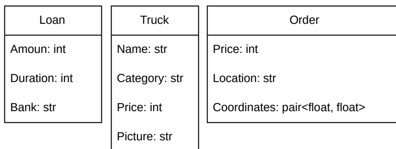
Рисунок 2.2 — Логічна схема
