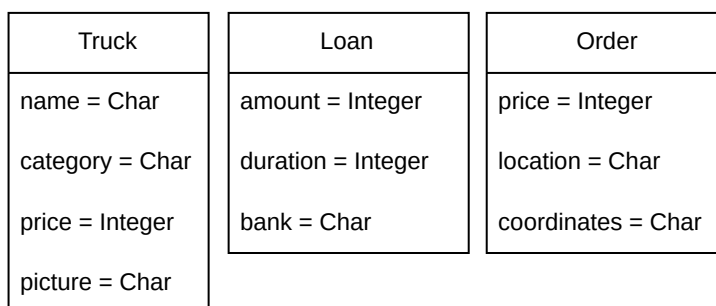
Рисунок 2.3 — Фізична схема
