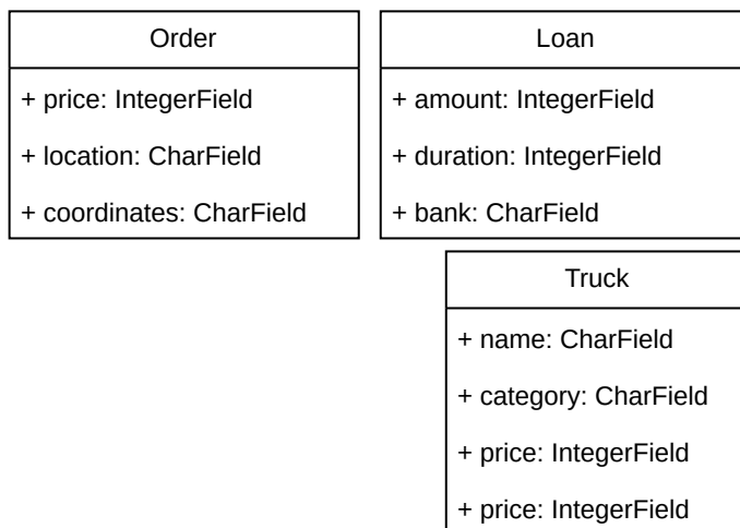
Рисунок 3.4 - ER-діаграма
