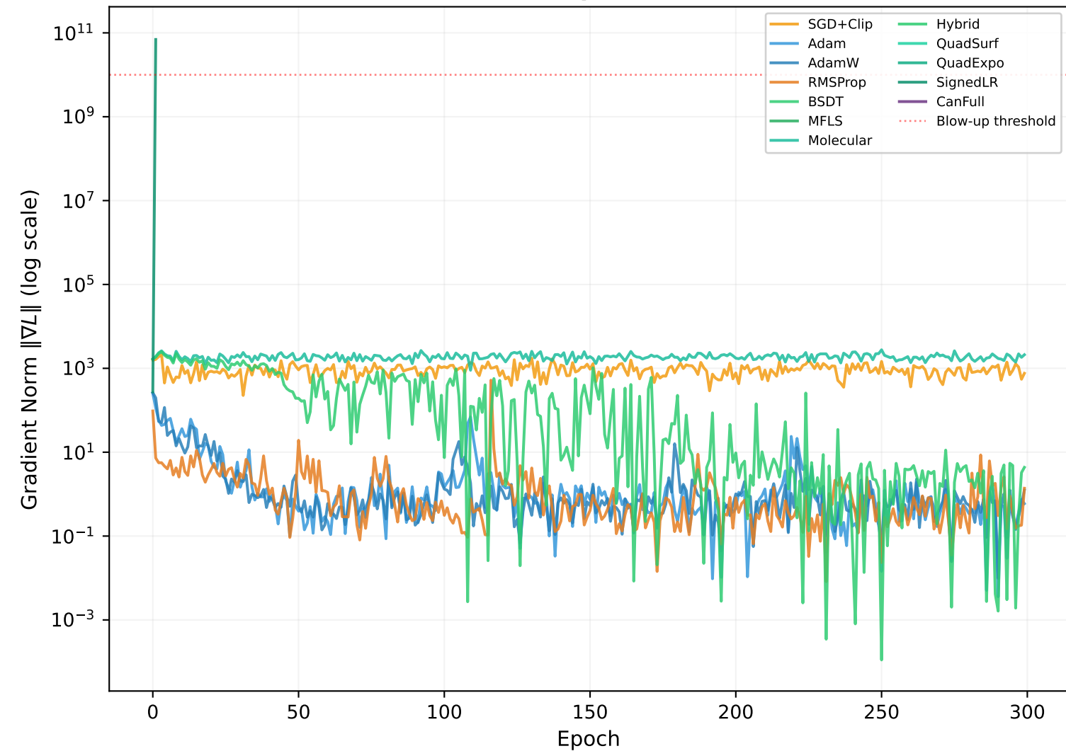
(b) Gradient Norm: Explosion vs Stabilisation
