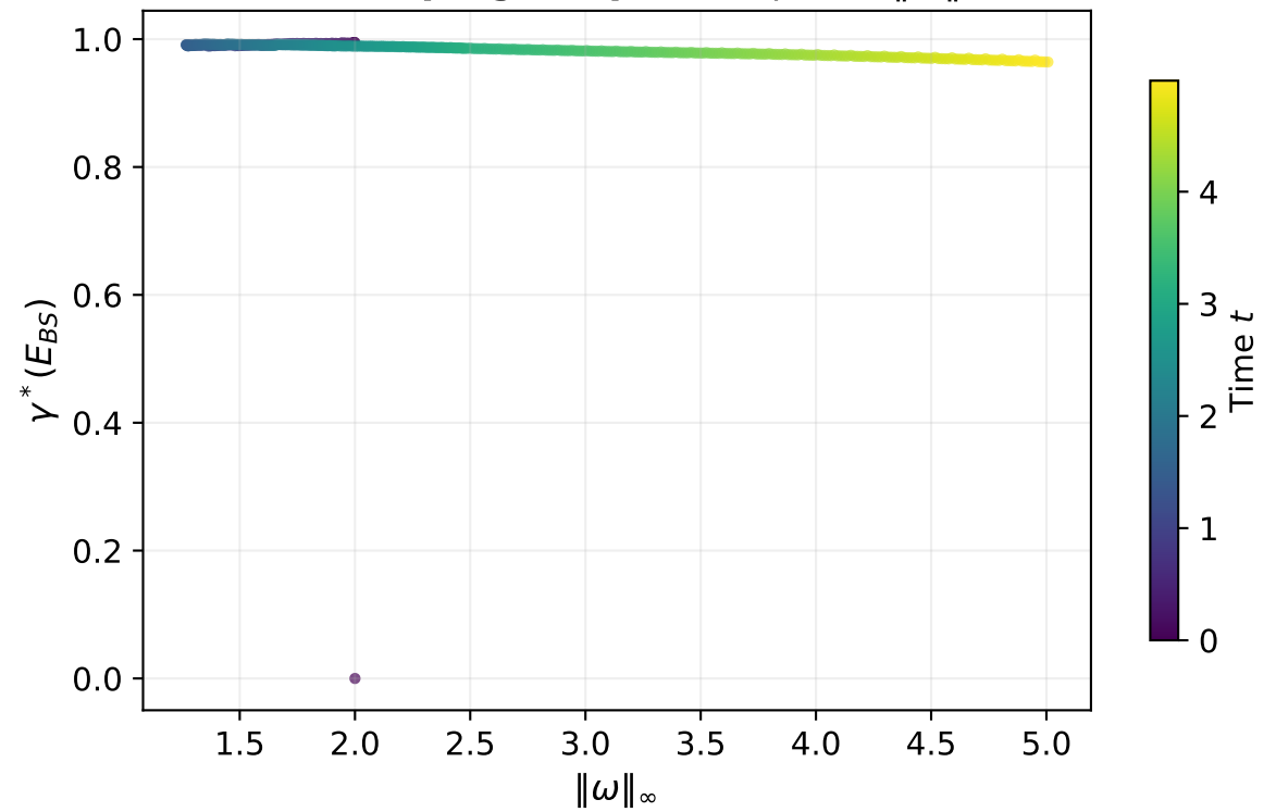
(d) Damping Response: \gamma^* vs \|\omega\|_\infty
