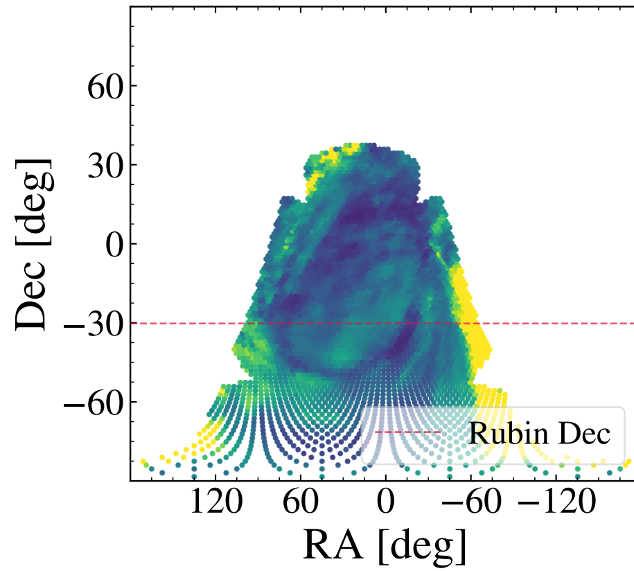
HEALPix RA / Dec
