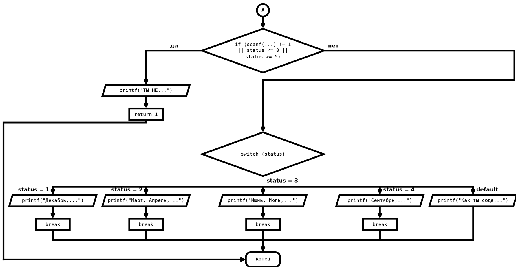
Рисунок 11: Блок-схема программы к заданию № 4 — лист 2
