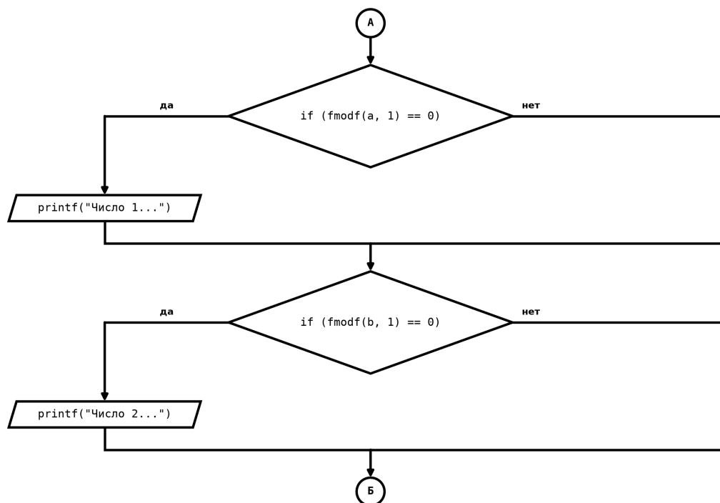
Рисунок 7: Блок-схема программы к заданию № 3 — лист 2; соединители «А» и «Б» связывают листы
