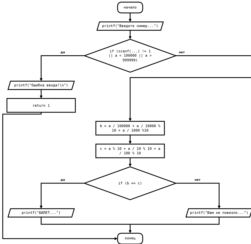
Рисунок 4: Блок-схема программы к заданию № 2
