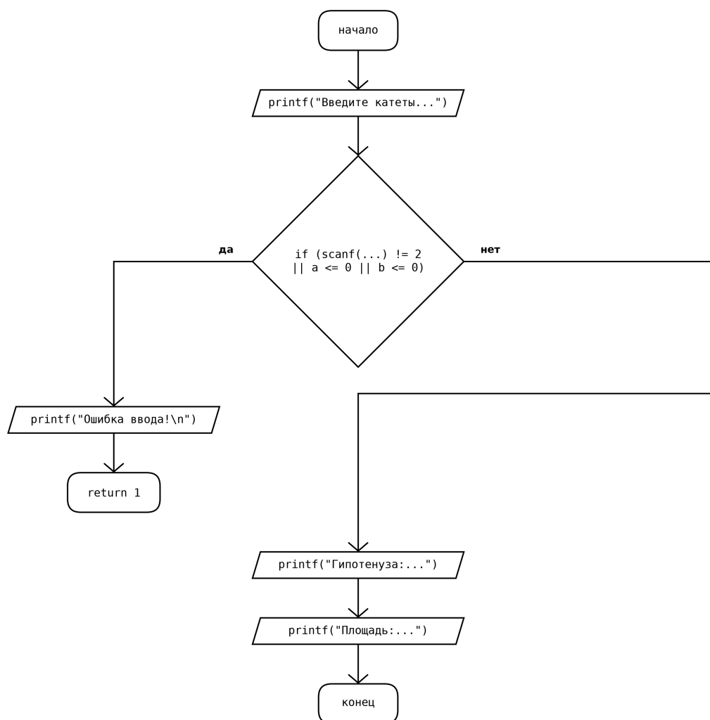
Рисунок 2 – Блок-схема программы к заданию № 1
