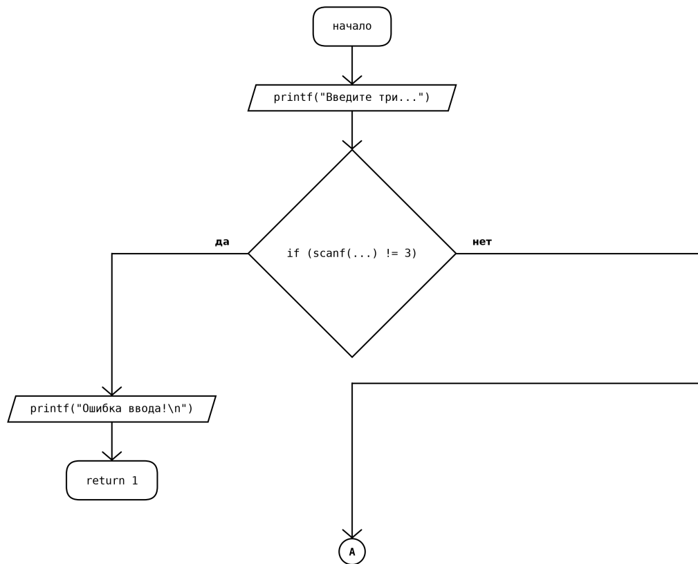
Рисунок 6 – Блок-схема программы к заданию № 3
