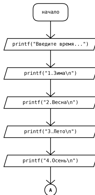
Рисунок 8 – Блок-схема программы к заданию № 4 — лист 1: меню
