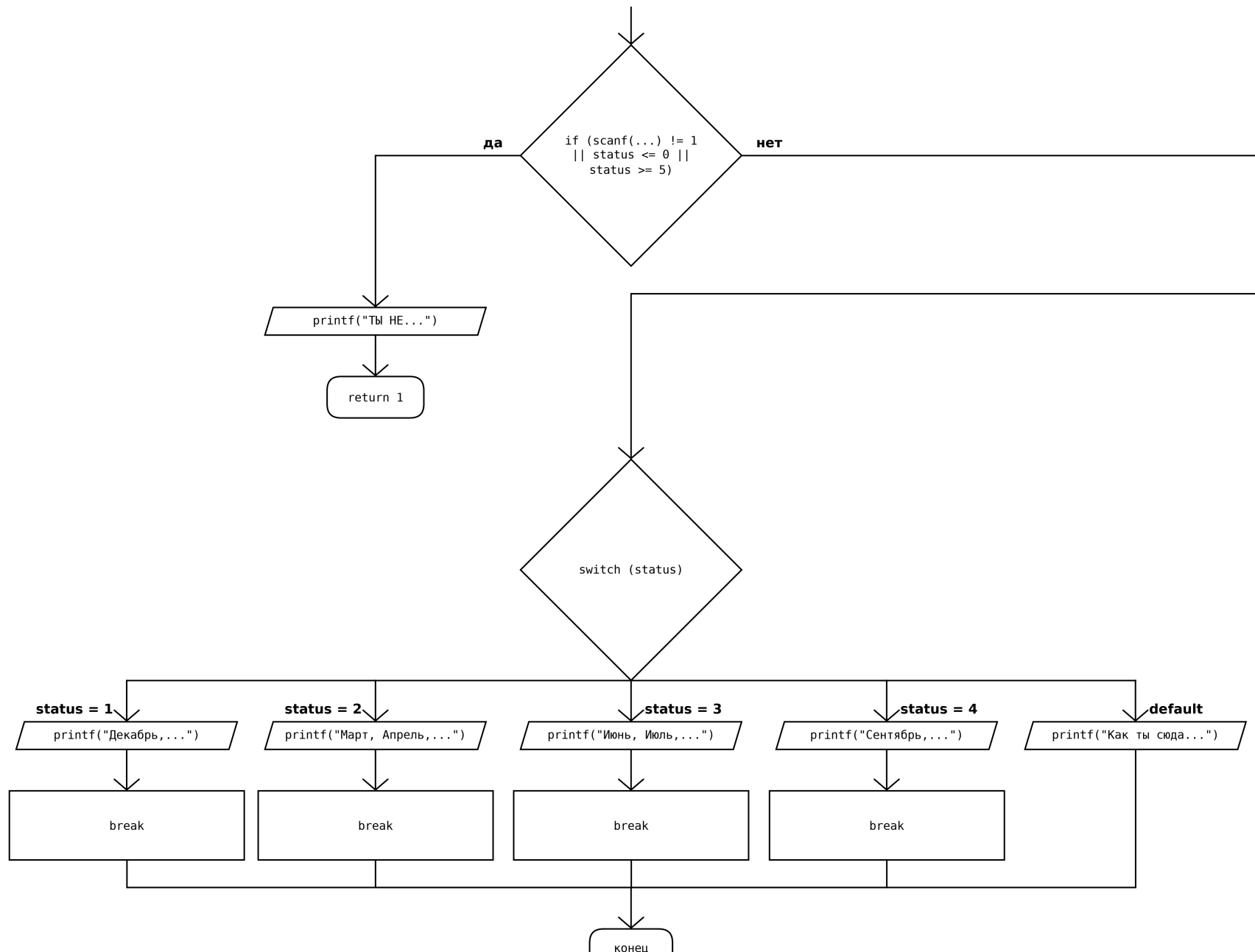
Рисунок 9 – Блок-схема программы к заданию № 4 — лист 2: выбор сезона
