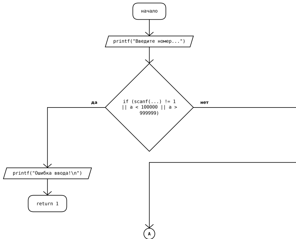
Рисунок 4 – Блок-схема программы к заданию № 2
