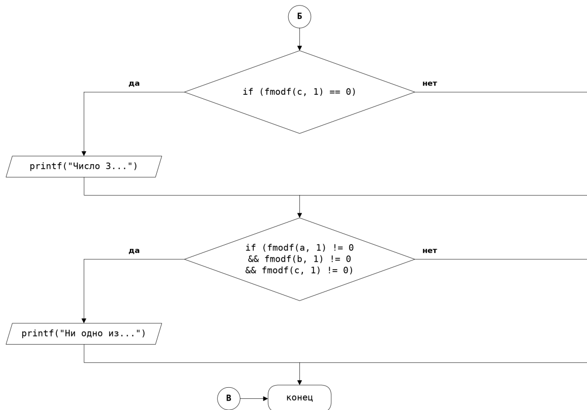
Рисунок 8 – Блок-схема программы к заданию № 3 — лист 3
