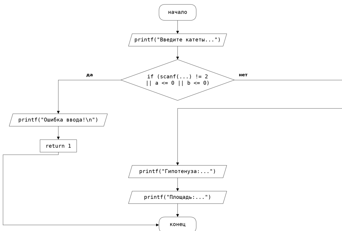
Рисунок 2 – Блок-схема программы к заданию № 1
