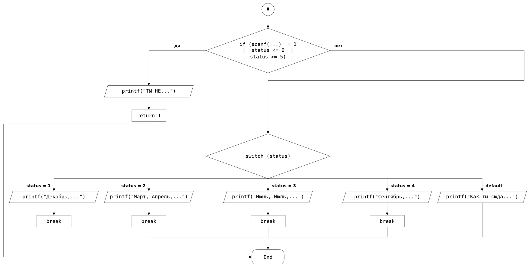
Рисунок 11 – Блок-схема программы к заданию № 4 — лист 2: проверка ввода и выбор сезона
