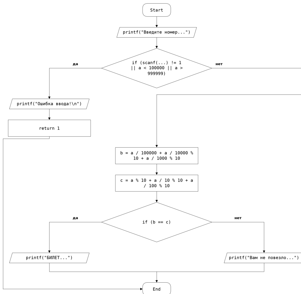
Рисунок 4 – Блок-схема программы к заданию № 2
