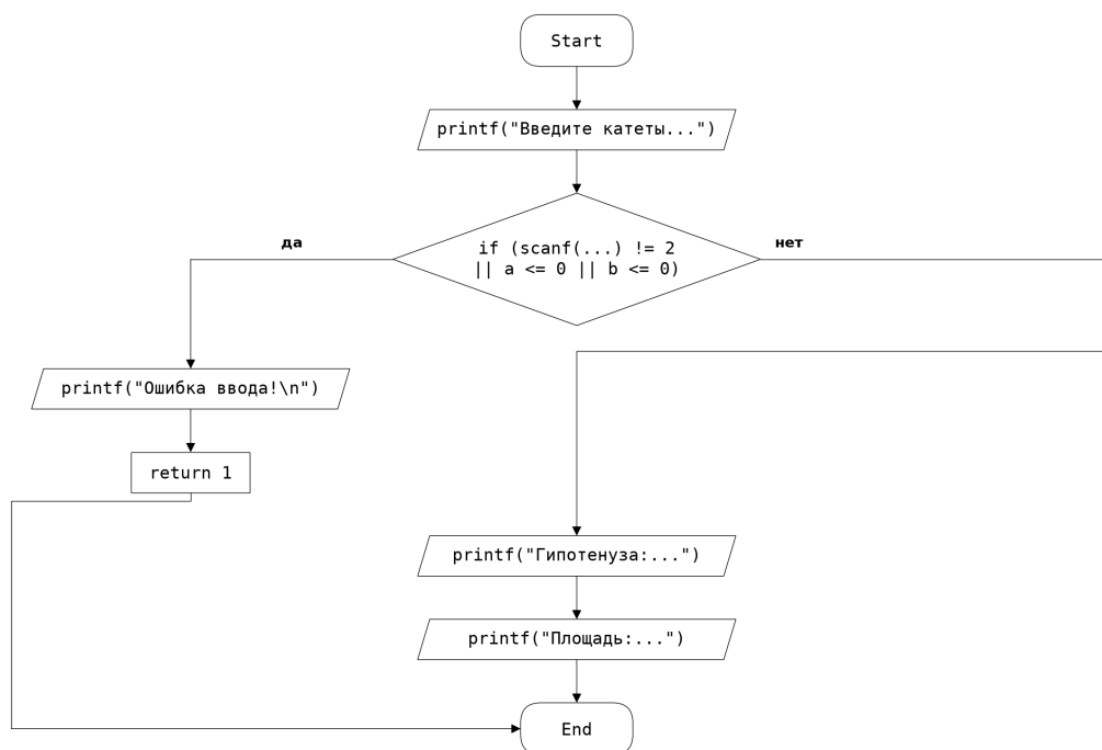
Рисунок 2 – Блок-схема программы к заданию № 1
