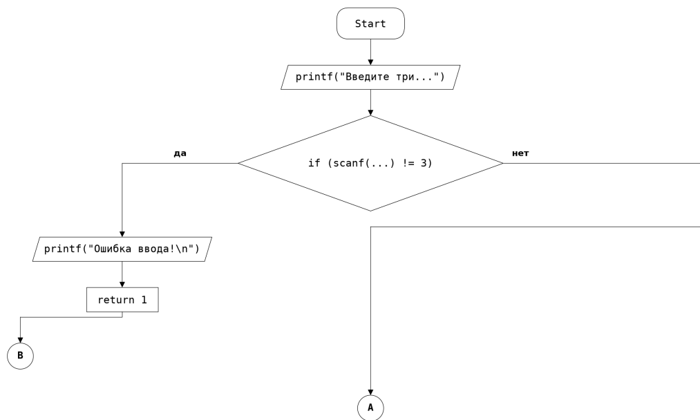
Рисунок 6 – Блок-схема программы к заданию № 3 — лист 1
