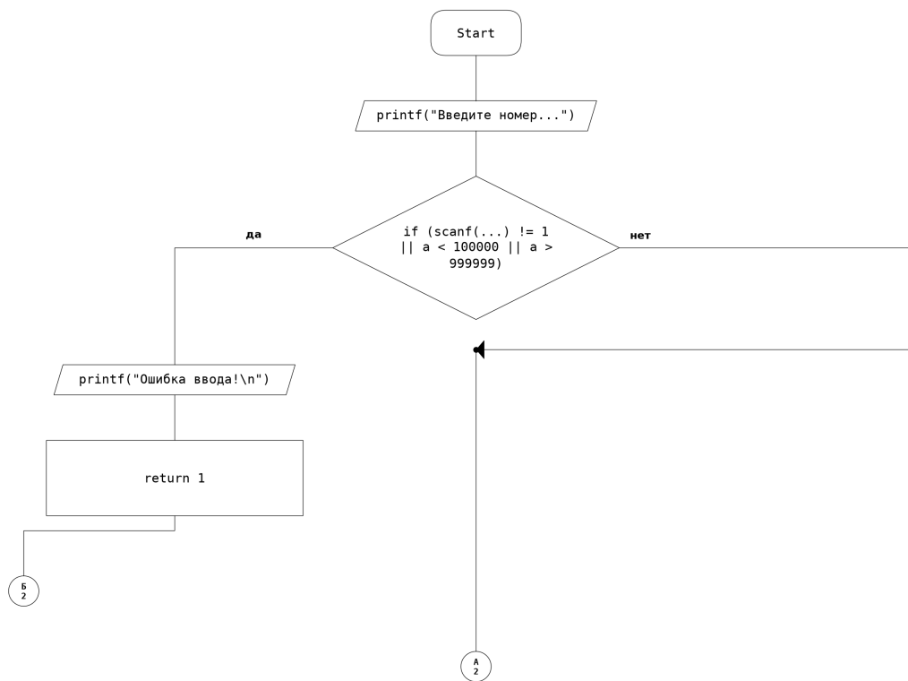
Рисунок 4 – Блок-схема программы к заданию № 2 — лист 1
