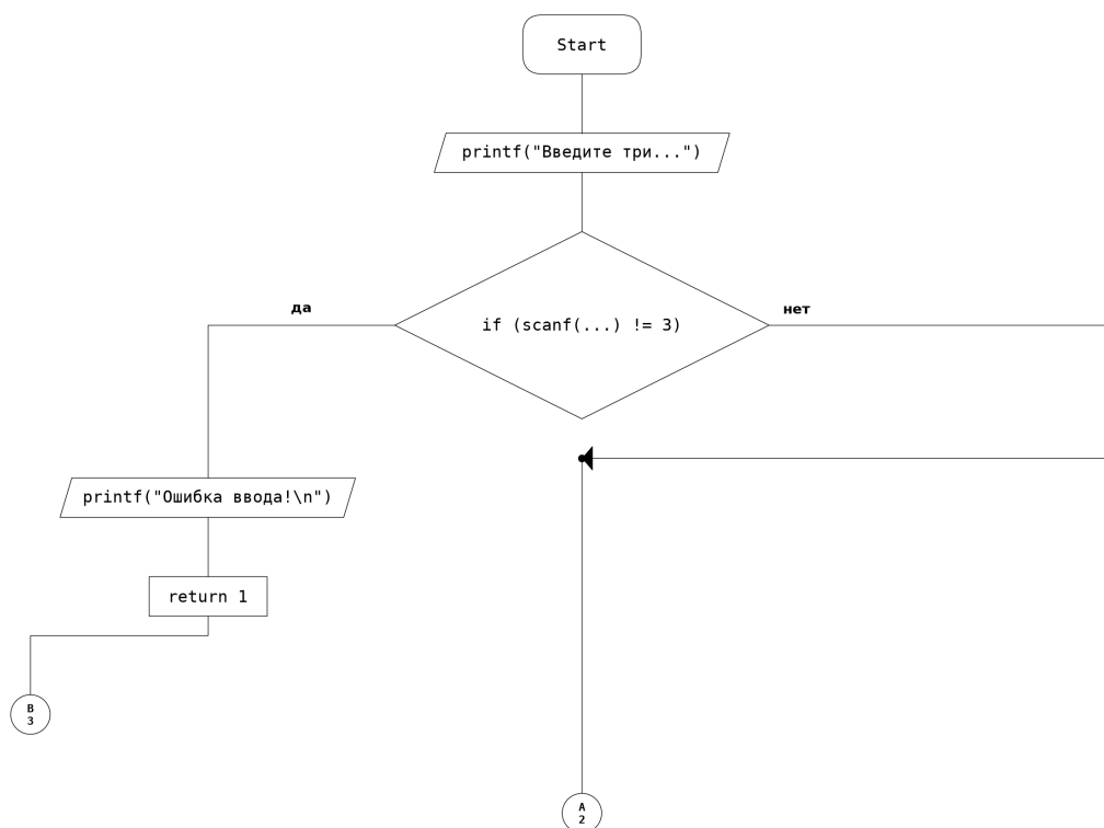
Рисунок 7 – Блок-схема программы к заданию № 3 — лист 1
