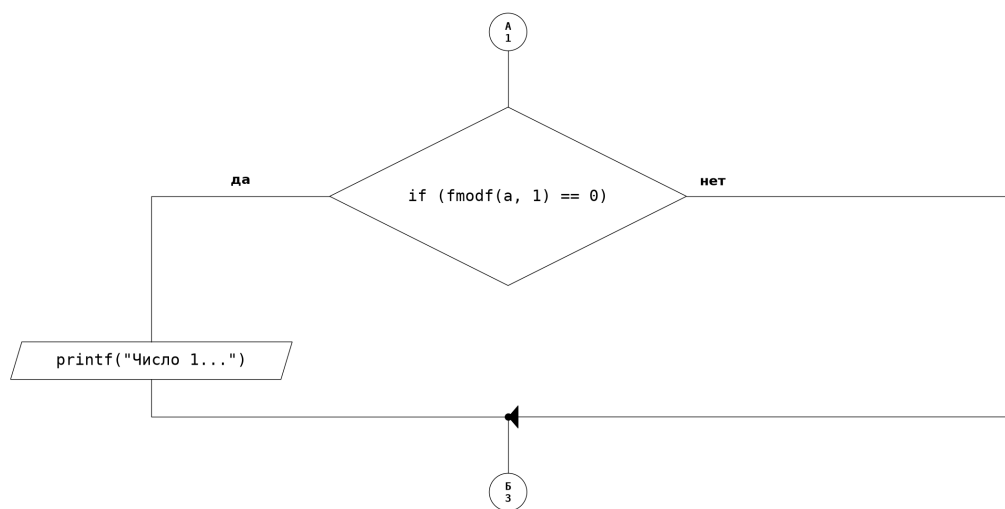
Рисунок 8 – Блок-схема программы к заданию № 3 — лист 2; соединители «А» и «Б» связывают листы
