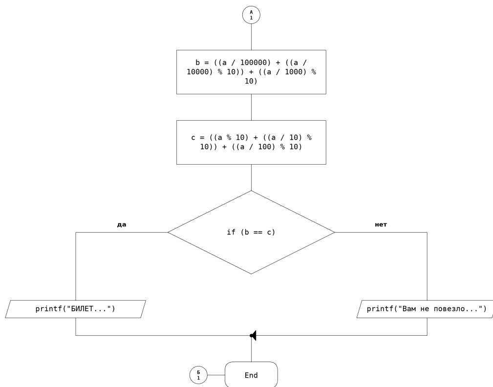
Рисунок 5 – Блок-схема программы к заданию № 2 — лист 2; соединители «А» и «Б» связывают листы
