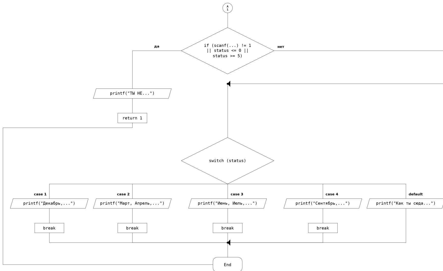
Рисунок 12 – Блок-схема программы к заданию № 4 — лист 2: выбор сезона
