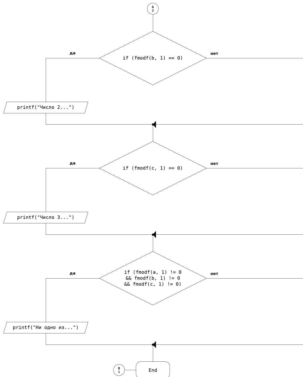
Рисунок 9 – Блок-схема программы к заданию № 3 — лист 3
