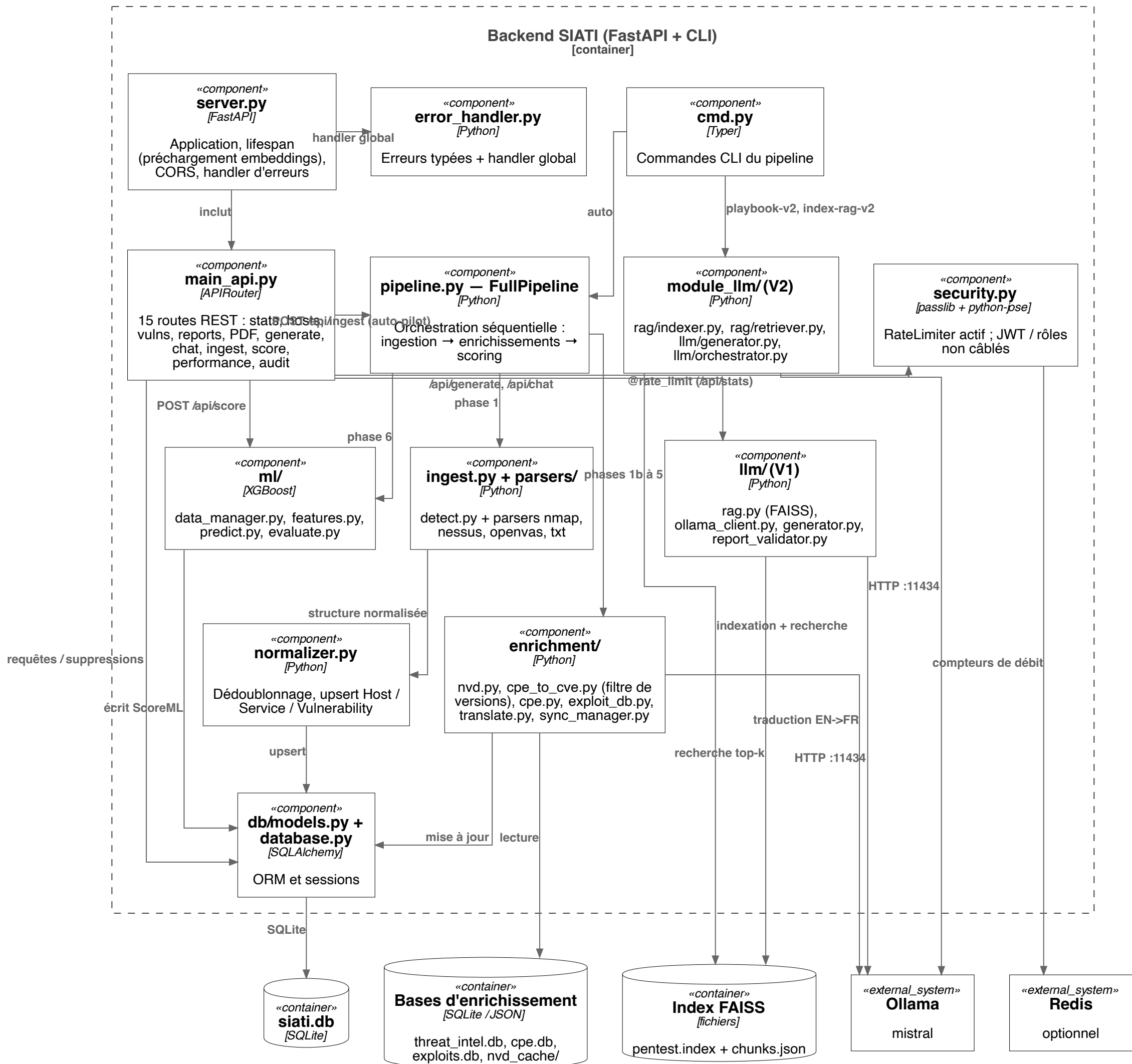
Diagramme C4 — Niveau 3 : Composants du backend SIATI
