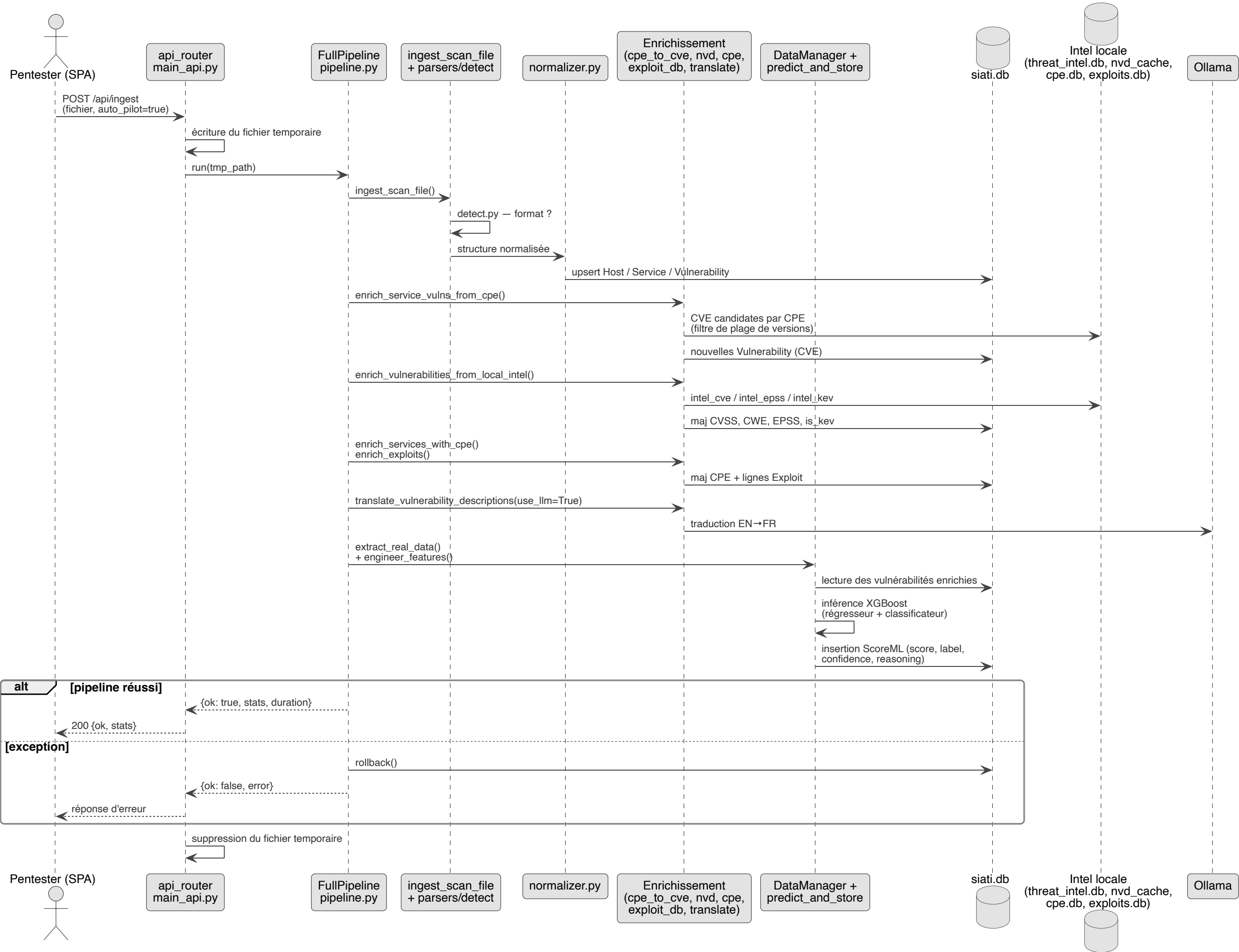
Diagramme de séquence — POST /api/ingest (mode auto-pilot)
