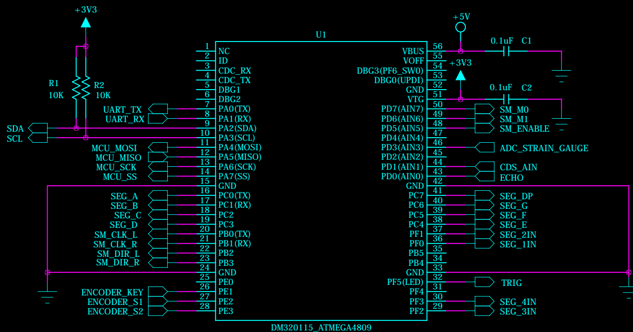
MCU(ATmega4809)
