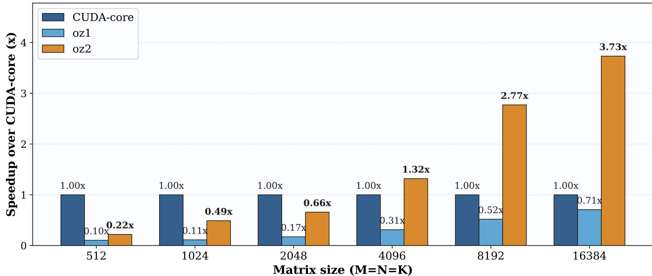
INT32 GEMM speedup vs CUDA-core per size (op=NN)
