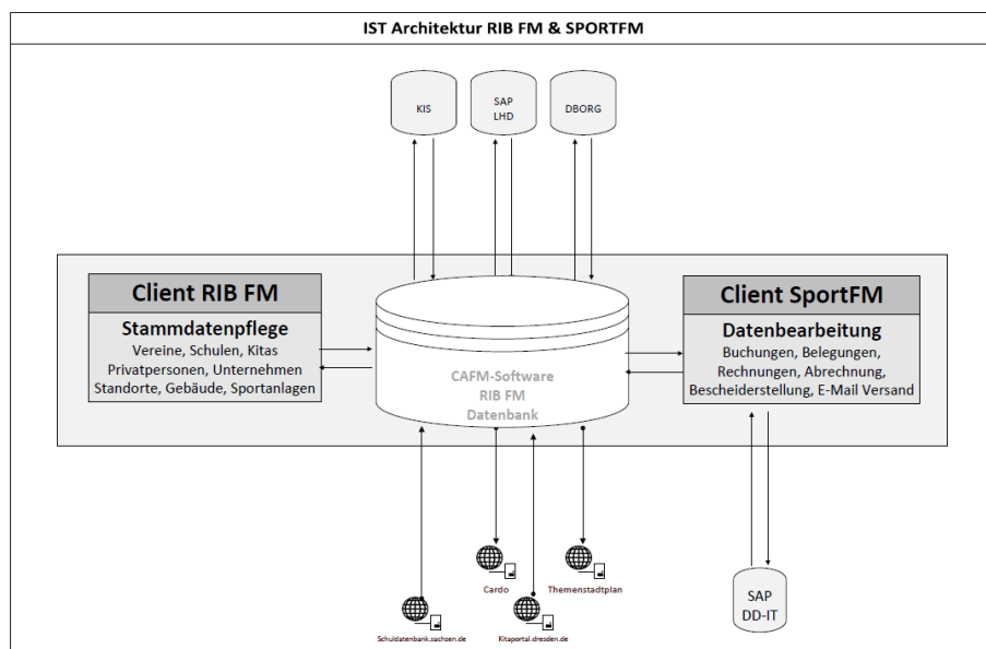
Abbildung 21: IST-Systemarchitektur RIB FM und SportFM
