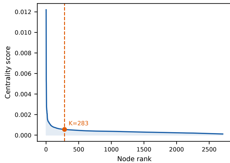
Citeseer x PageRank
