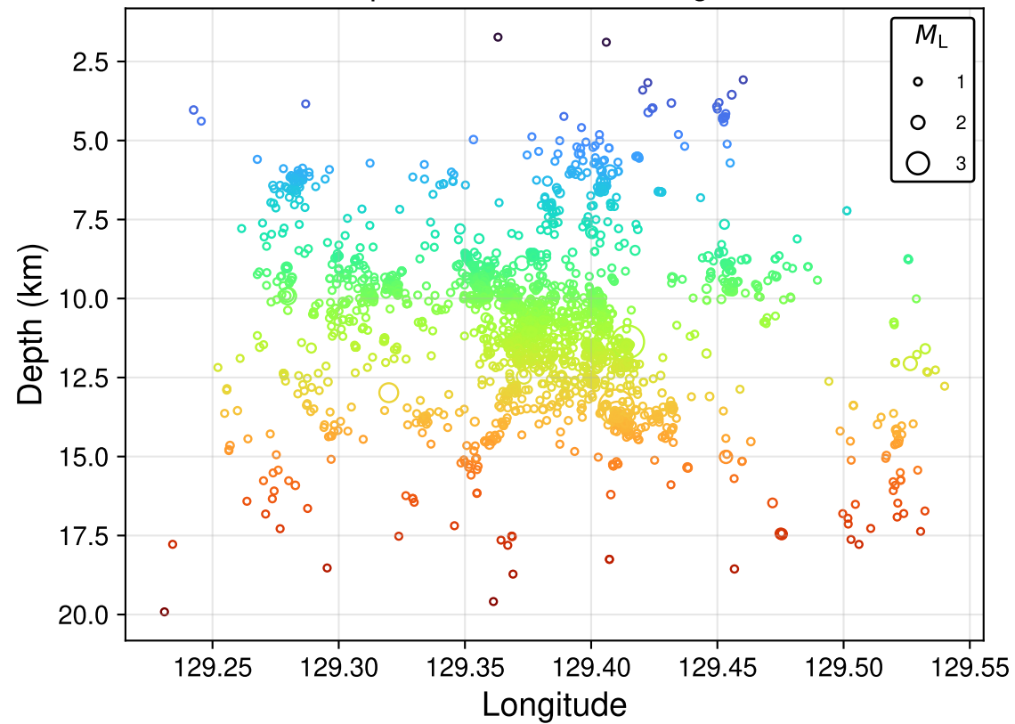
Depth section across longitude
