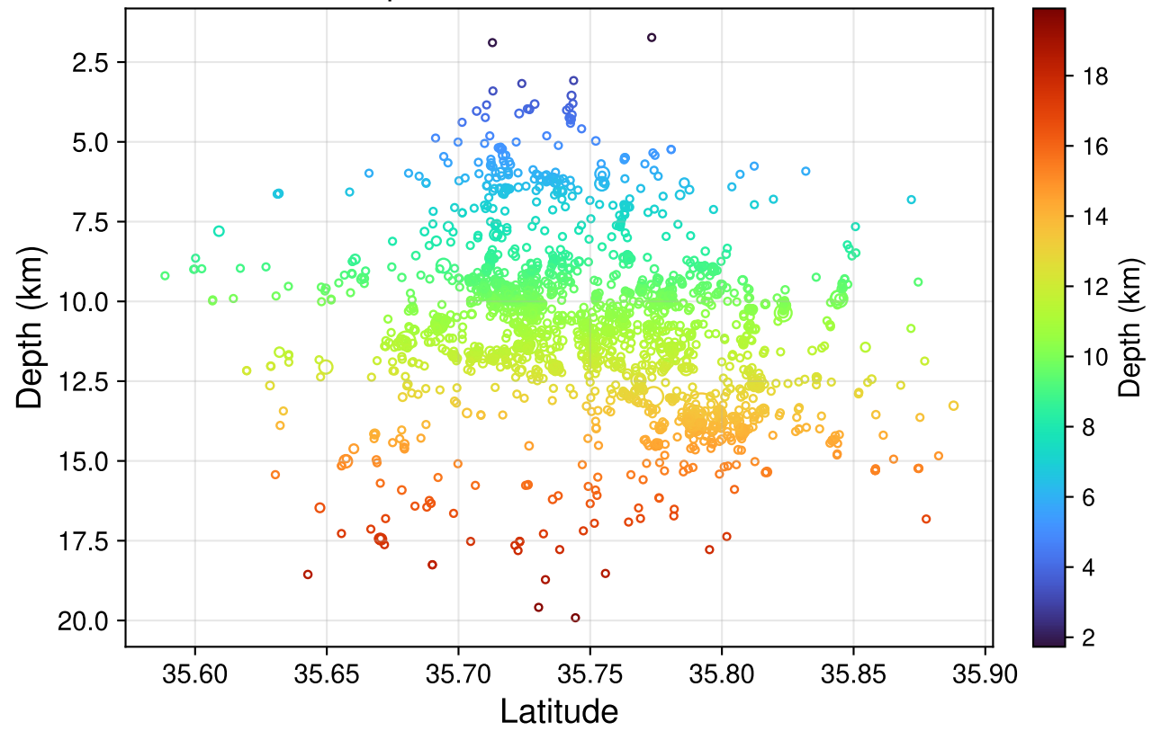
Depth section across latitude
