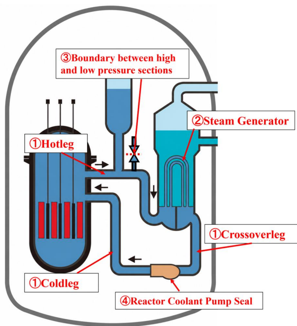
図1 原子炉冷却材が流出する主な場所 (3)
