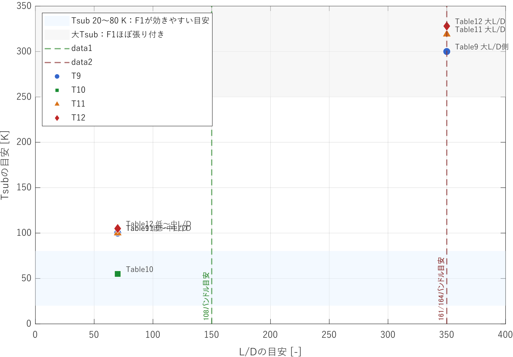
図2 L/Dを大きくするとTsubも大きくなる問題
