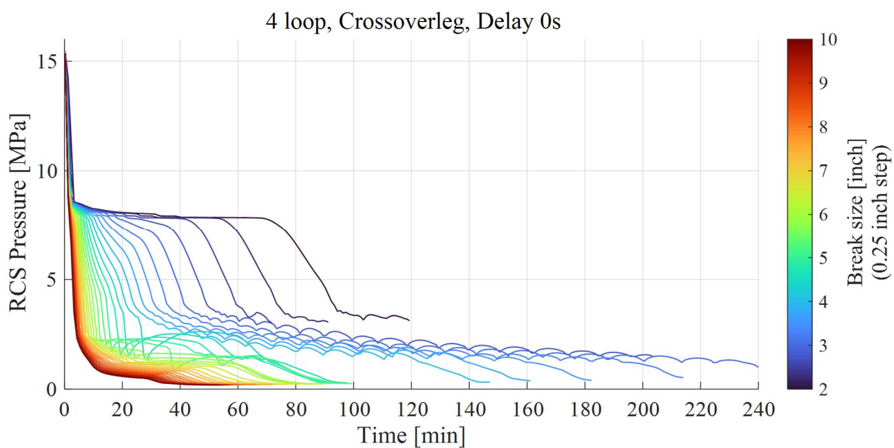
図 8 RCS 圧力の時間変化(クロスオーバーレグ破断, 4 ループ)
