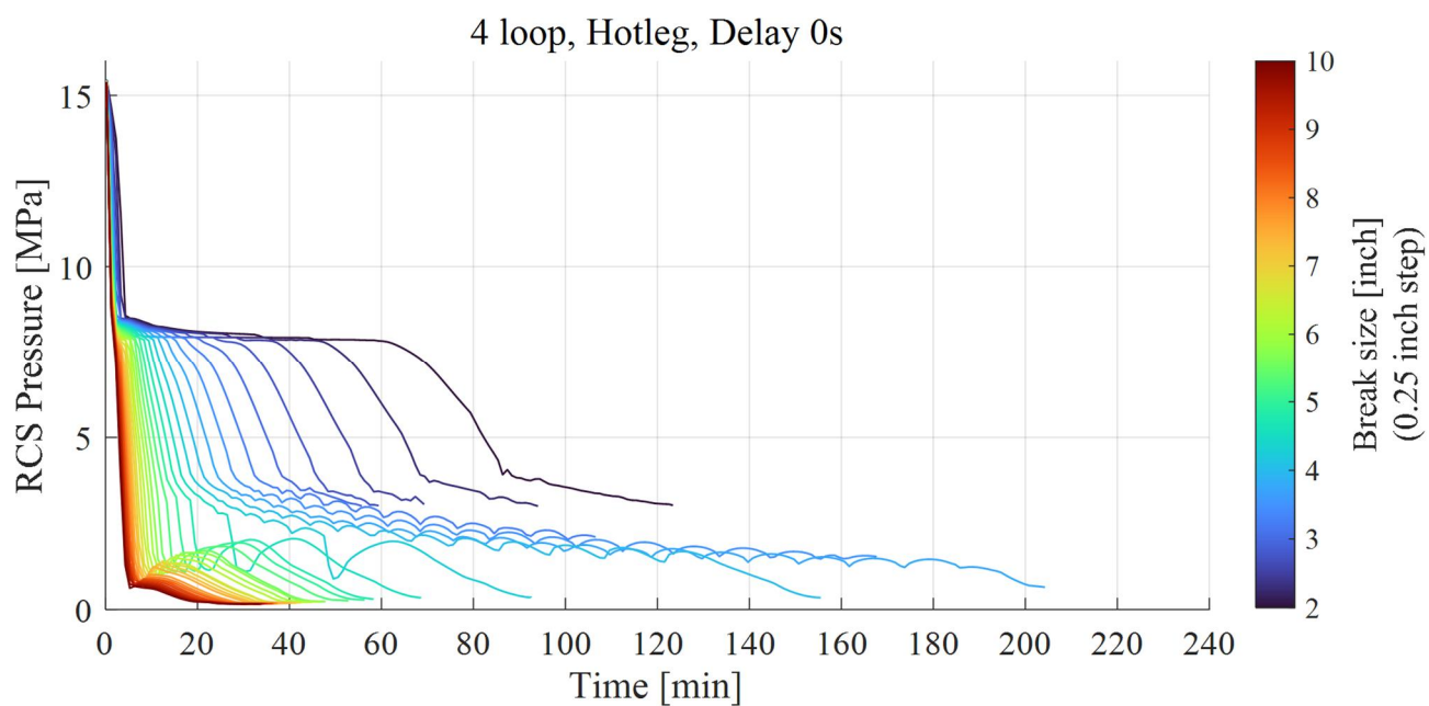
図 7 RCS 圧力の時間変化(ホットレグ破断, 4 ループ)
