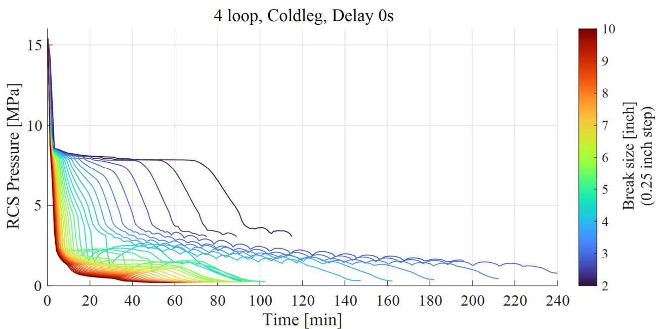
図 9 RCS 圧力の時間変化(コールドレグ破断, 4 ループ)
