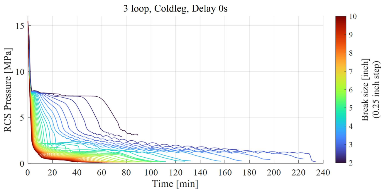
図 6 RCS 圧力の時間変化(コールドレグ破断, 3 ループ)
