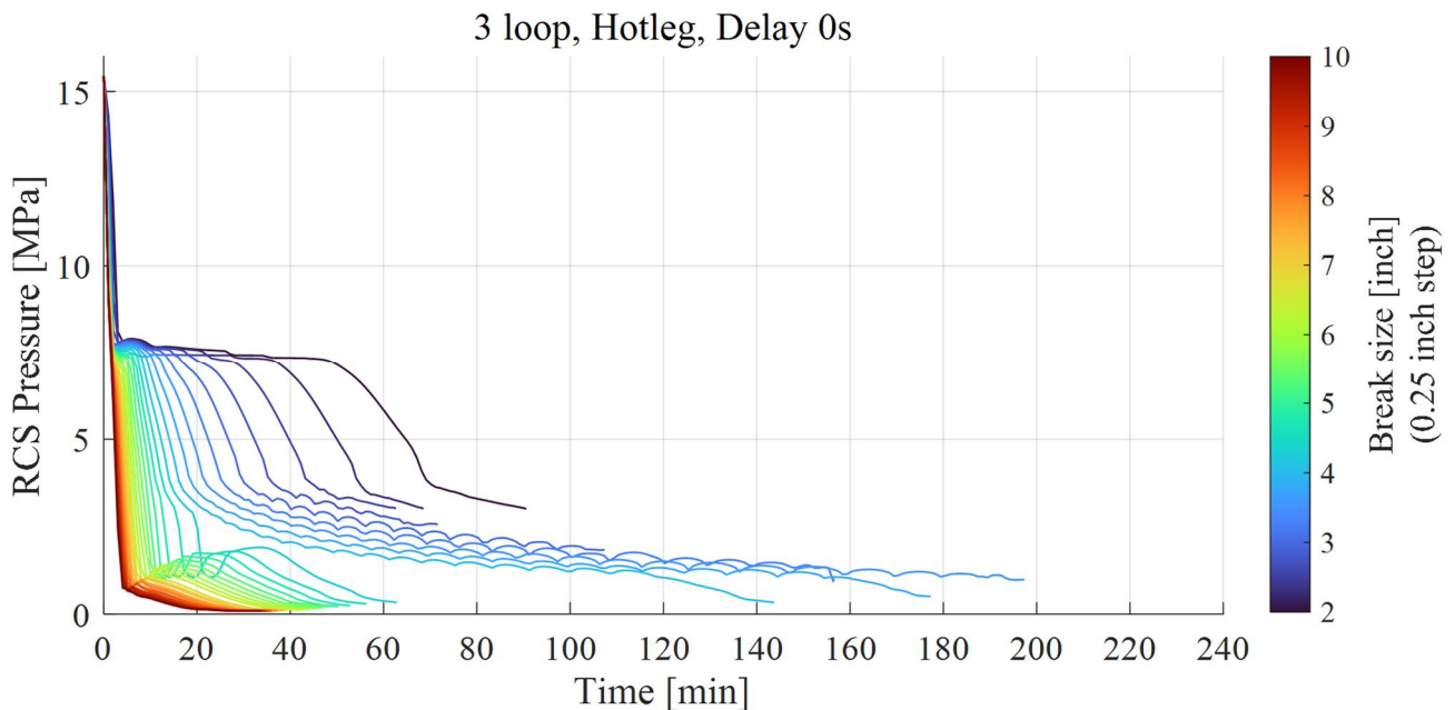
図 4 RCS 圧力の時間変化(ホットレグ破断, 3 ループ)
