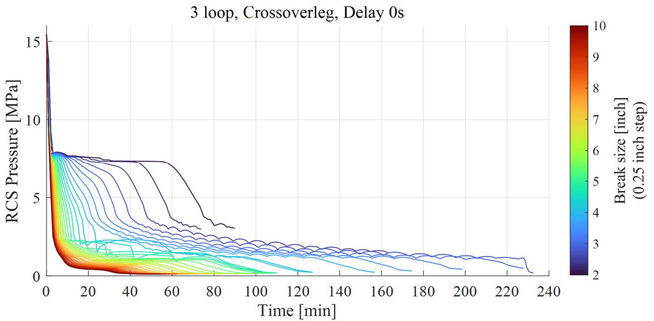
図 5 RCS 圧力の時間変化(クロスオーバーレグ破断, 3 ループ)
