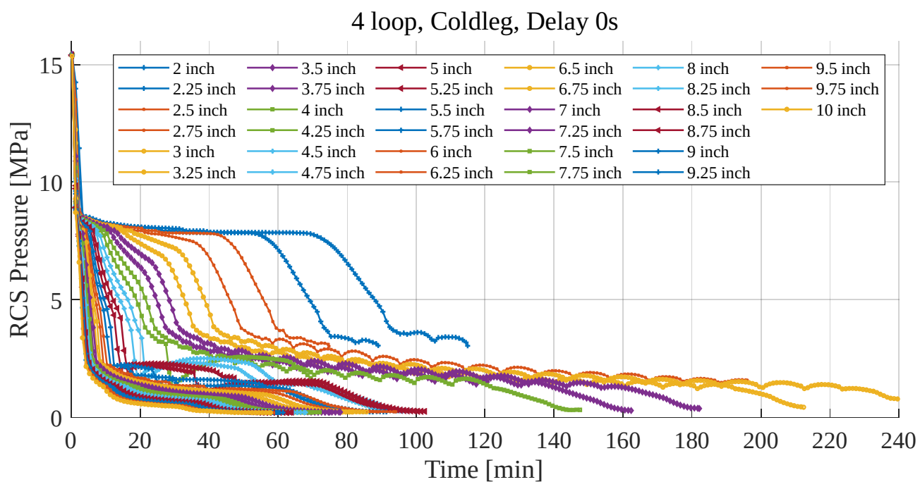
図 17 RCS 圧力の時間変化(コールドレグ破断, 4 ループ)
