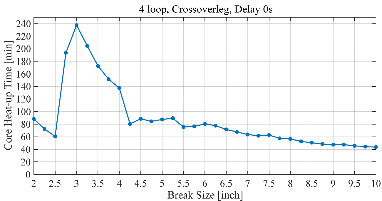
図 16 破断口径と炉心過熱時間の関係(クロスオーバーレグ破断, 4 ループ)
