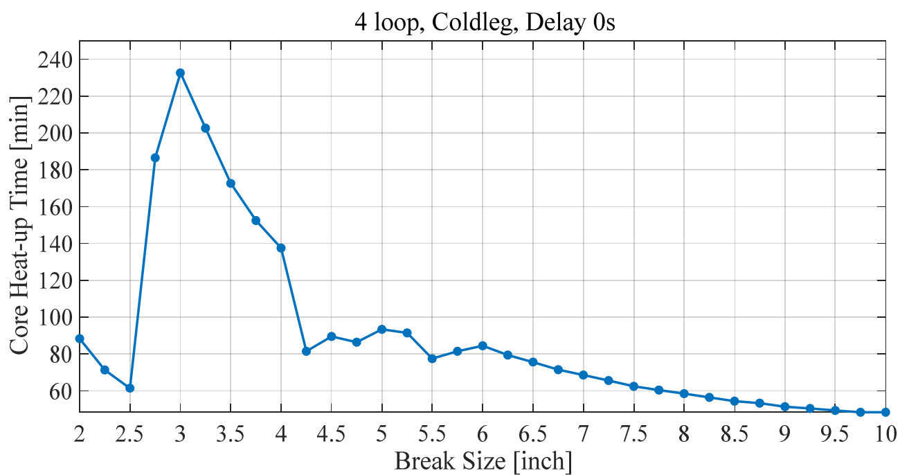
図 18 破断口径と炉心過熱時間の関係(コールドレグ破断, 4 ループ)
