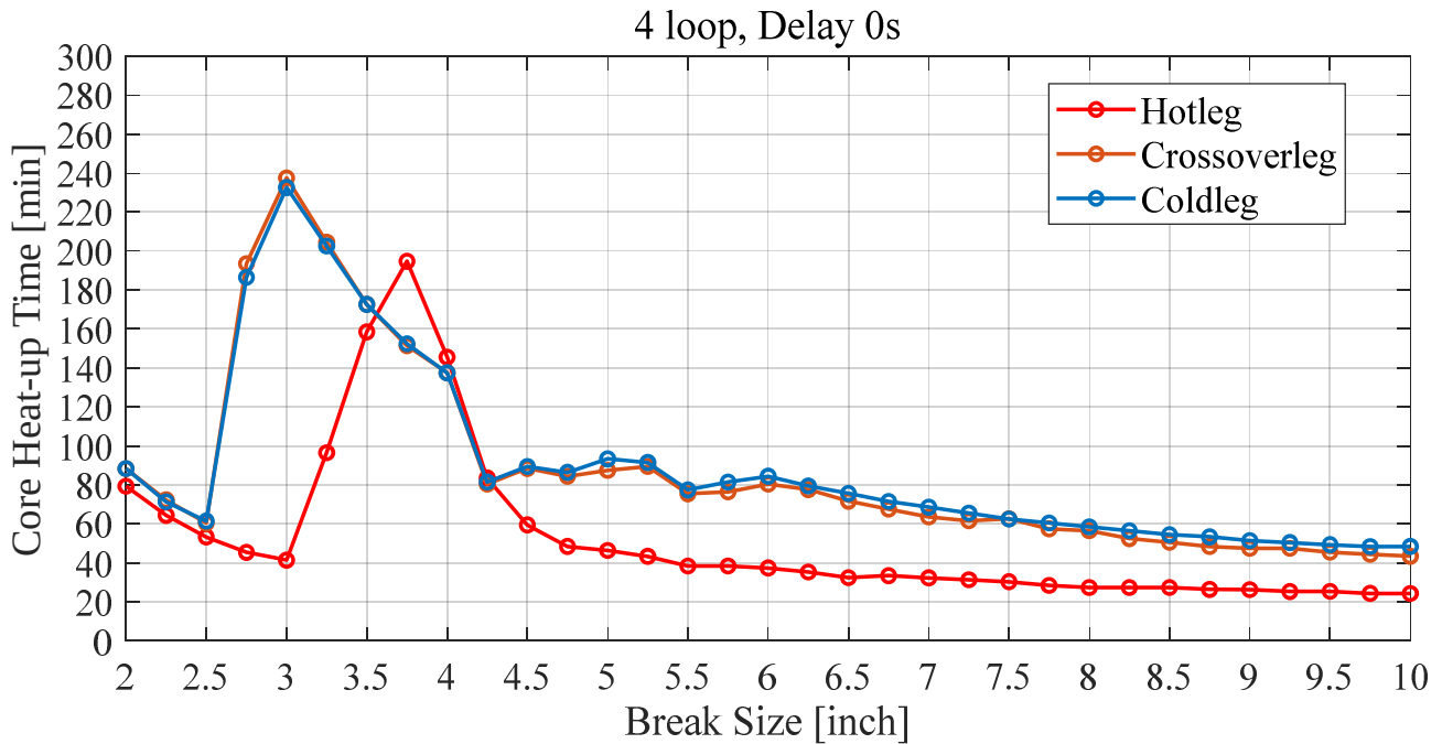
図 19 破断箇所別の炉心過熱時間の比較(4 ループ)
