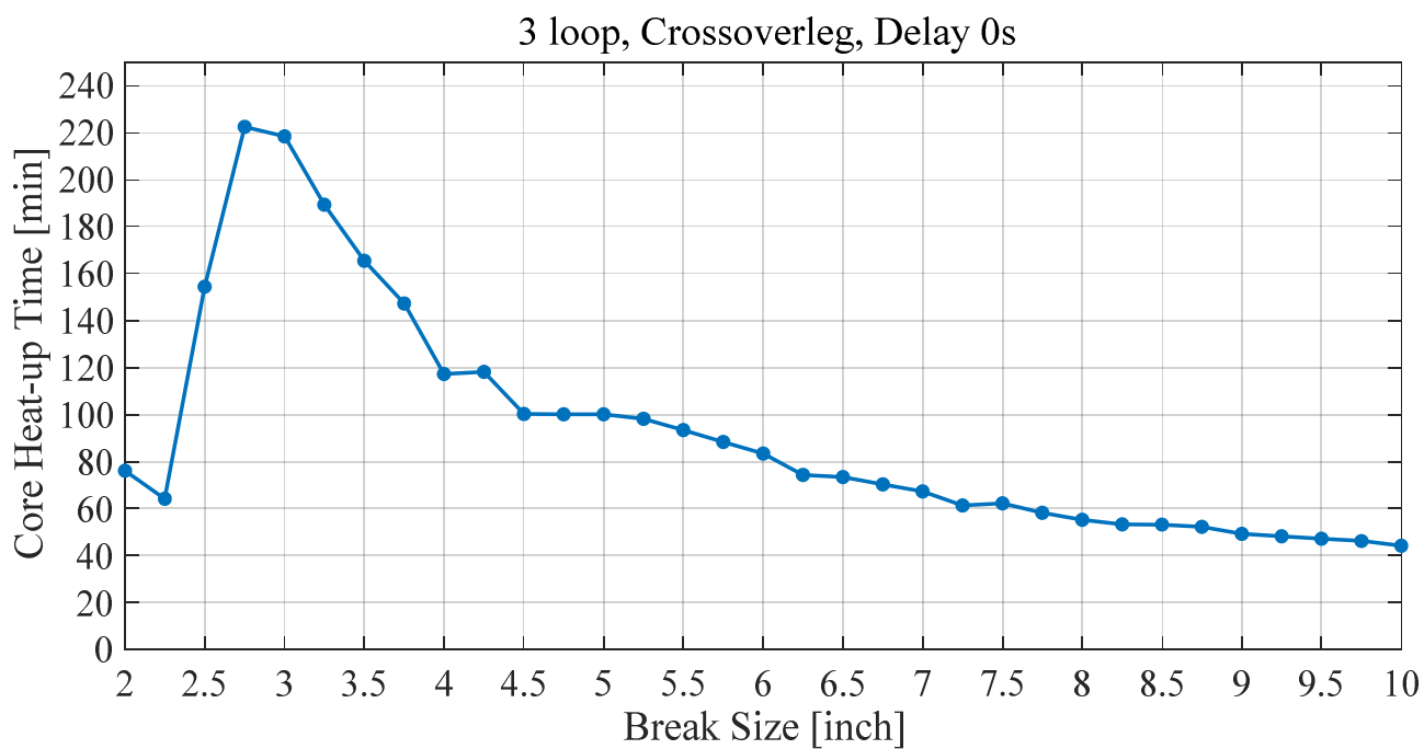
図 8 破断口径と炉心過熱時間の関係(クロスオーバーレグ破断, 3 ループ)
