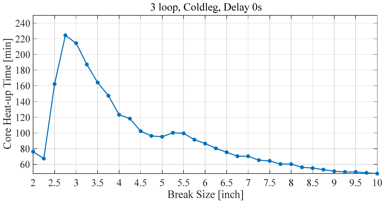
図 10 破断口径と炉心過熱時間の関係(コールドレグ破断, 3 ループ)
