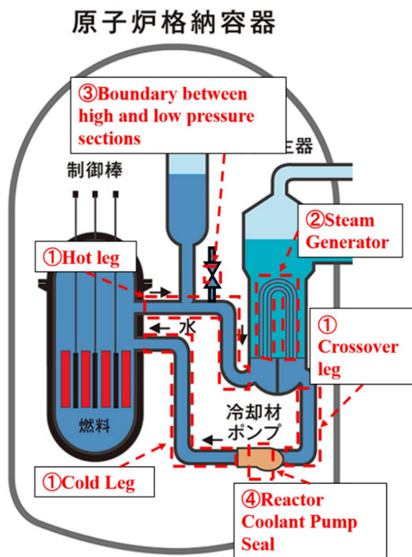
図1 原子炉冷却材が流出する主な場所(3)
