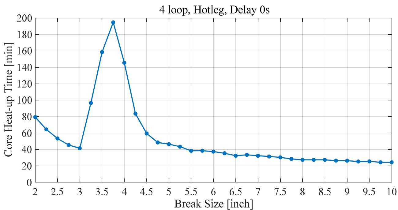
図 14 破断口径と炉心過熱時間の関係(ホットレグ破断, 4 ループ)
