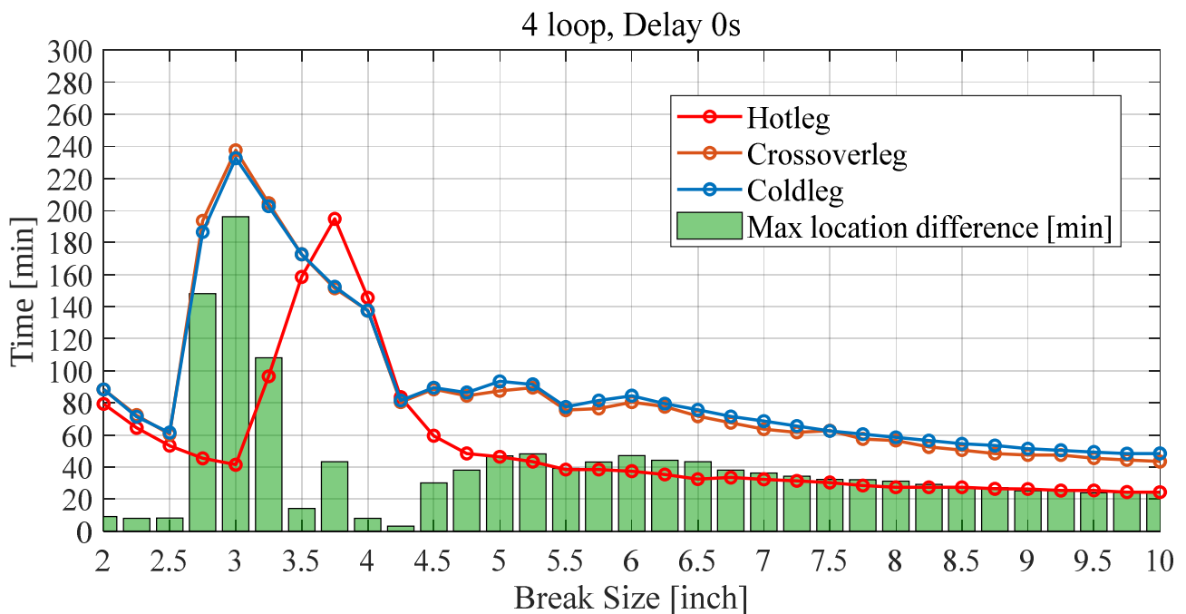
図 20 破断箇所別の炉心過熱時間および破断箇所間最大差の比較(4 ループ)
