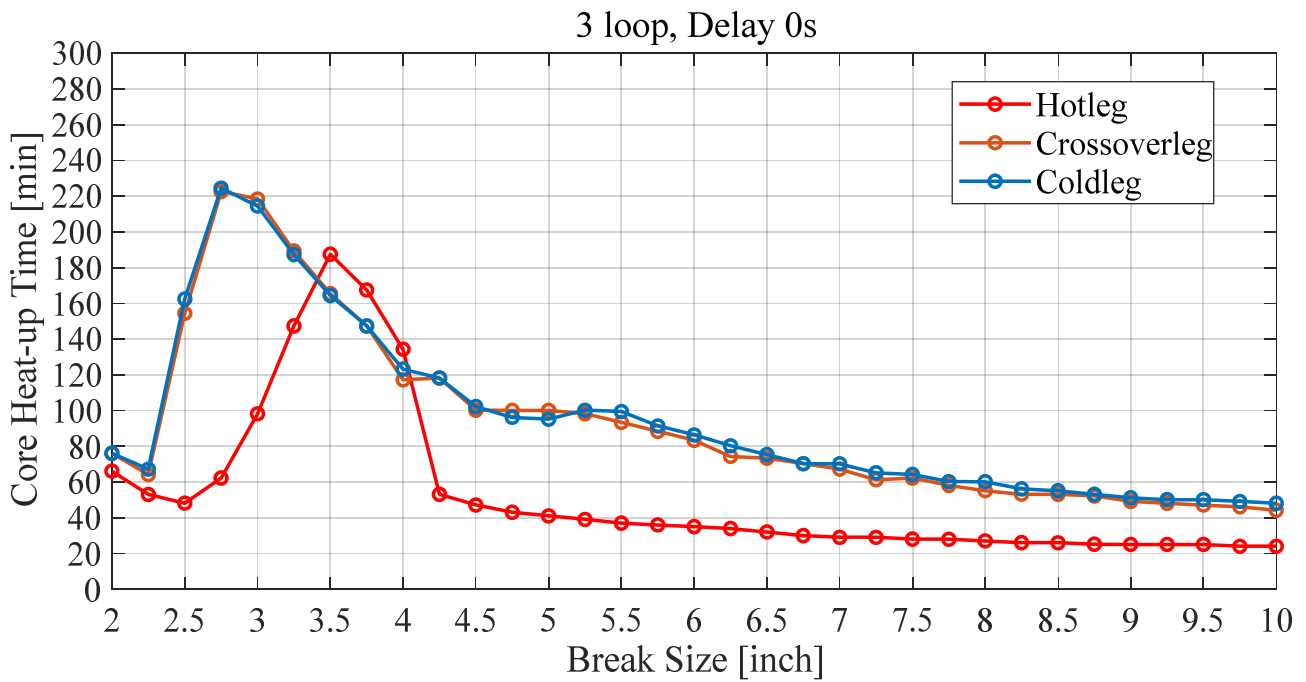
図 11 破断箇所別の炉心過熱時間の比較(3 ループ)
