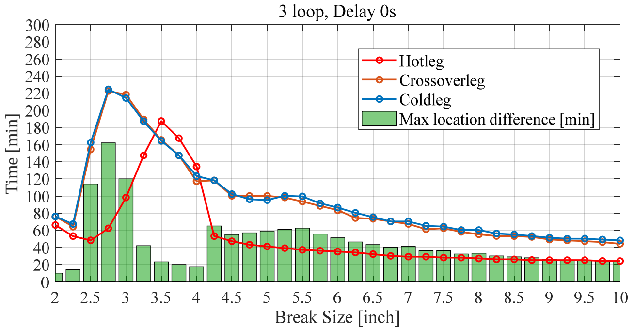
図 12 破断箇所別の炉心過熱時間および破断箇所間最大差の比較(3 ループ)
