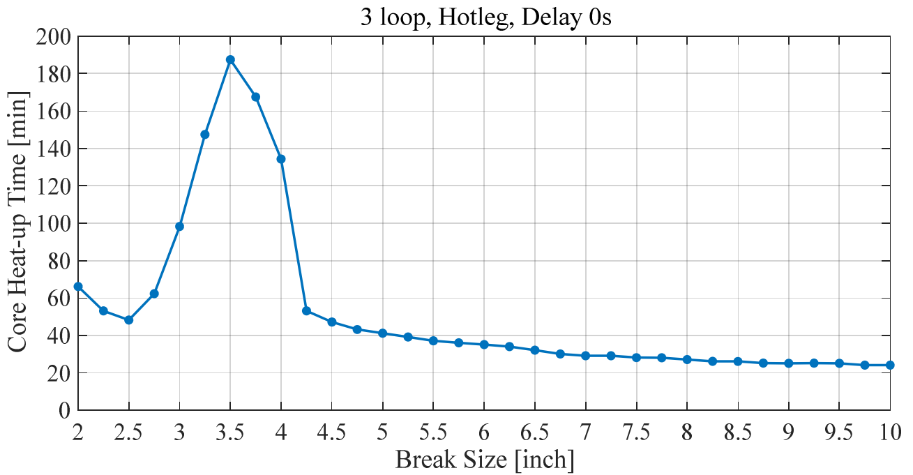
図 6 破断口径と炉心過熱時間の関係(ホットレグ破断, 3 ループ)
