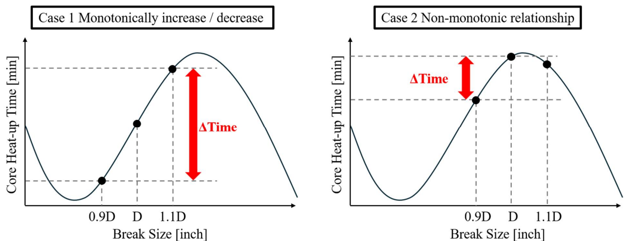
図 4 単調増加/単調減少，ピークをもつ場合の炉心過熱時間の評価方法
