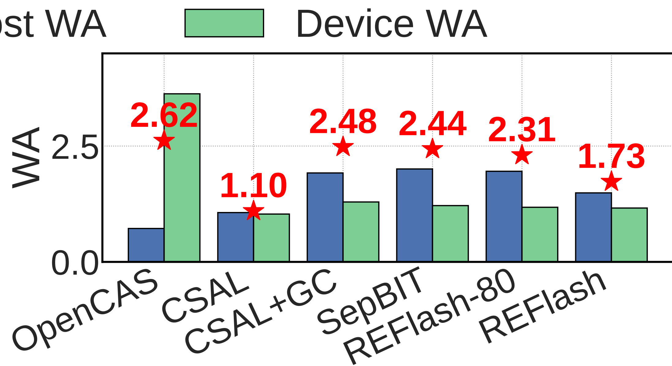
(b) YCSB-A
