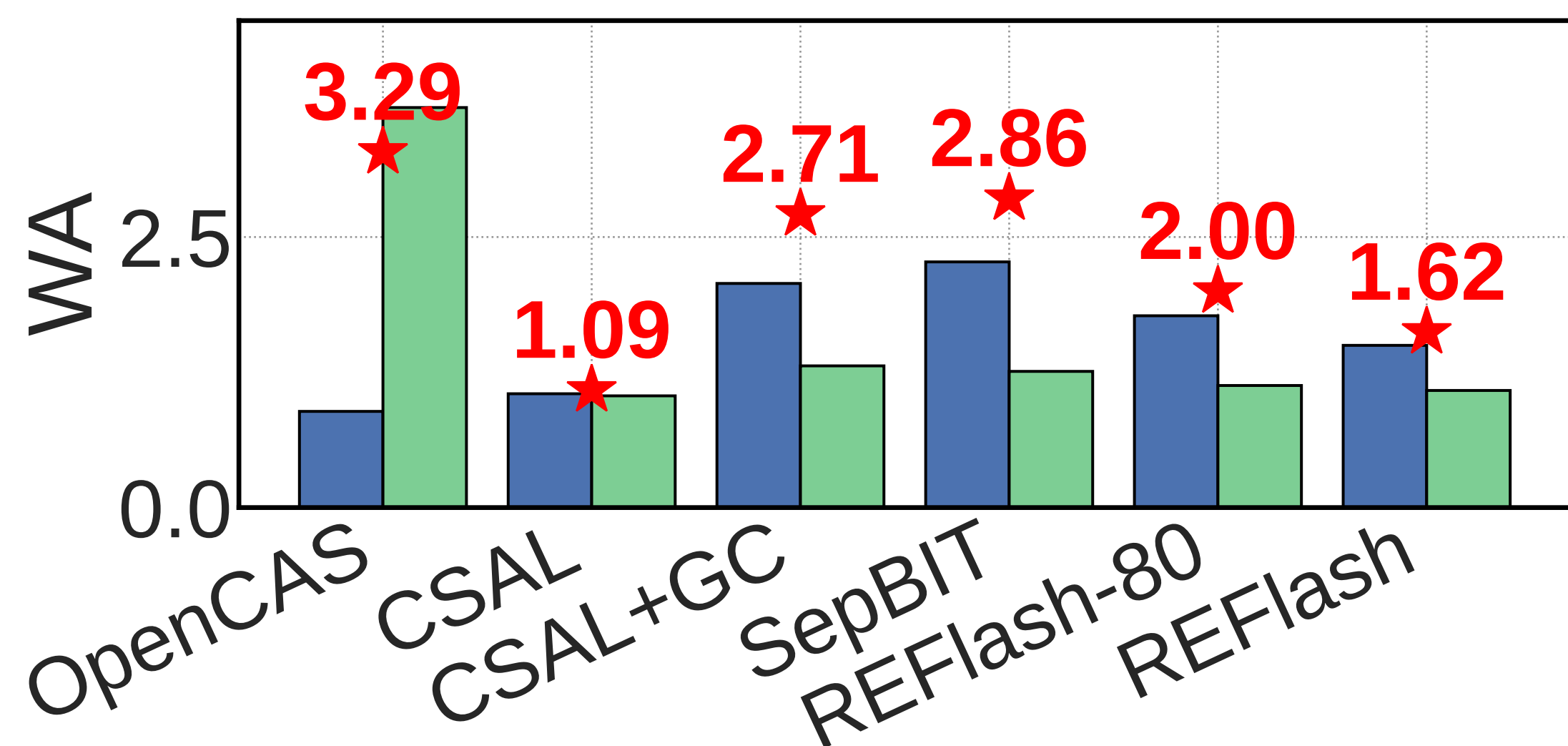
(d) Alibaba2
