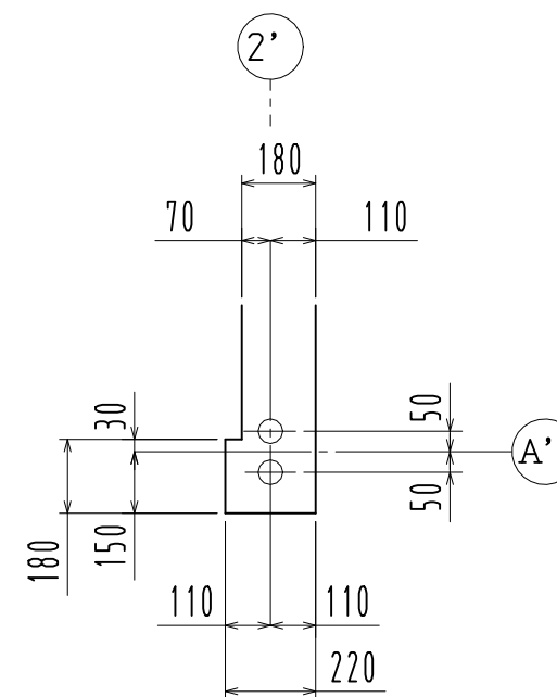
部分拡大図 1/20
