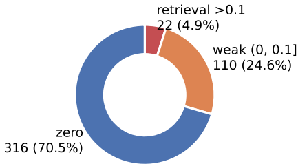
Qwen3-0.6B
