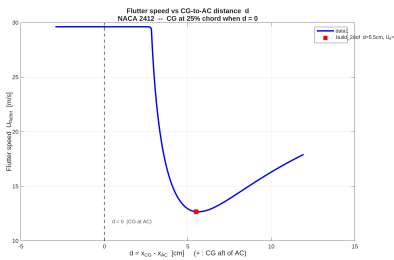
(b) 공력중심과 무게중심 사이 간격 d 에 따른 속도와 flutter boundary 사이의 관계
