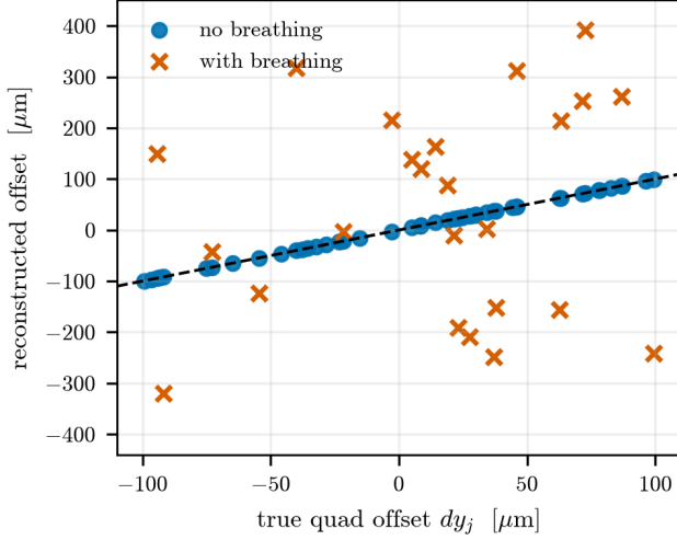
FIG. 7. Kuadrupol-başına gradyan modülasyonunun genlik olarak okunması: geri-çatılan ofsetlere karşı gerçek ofsetler. Optik nefes yapay olarak kaldırıldığında geri-çatma tamdır, ama nefes varken onunla ilişkisizdir — modülasyonla tutarlı olan nefes ortalamp azalmaz.
