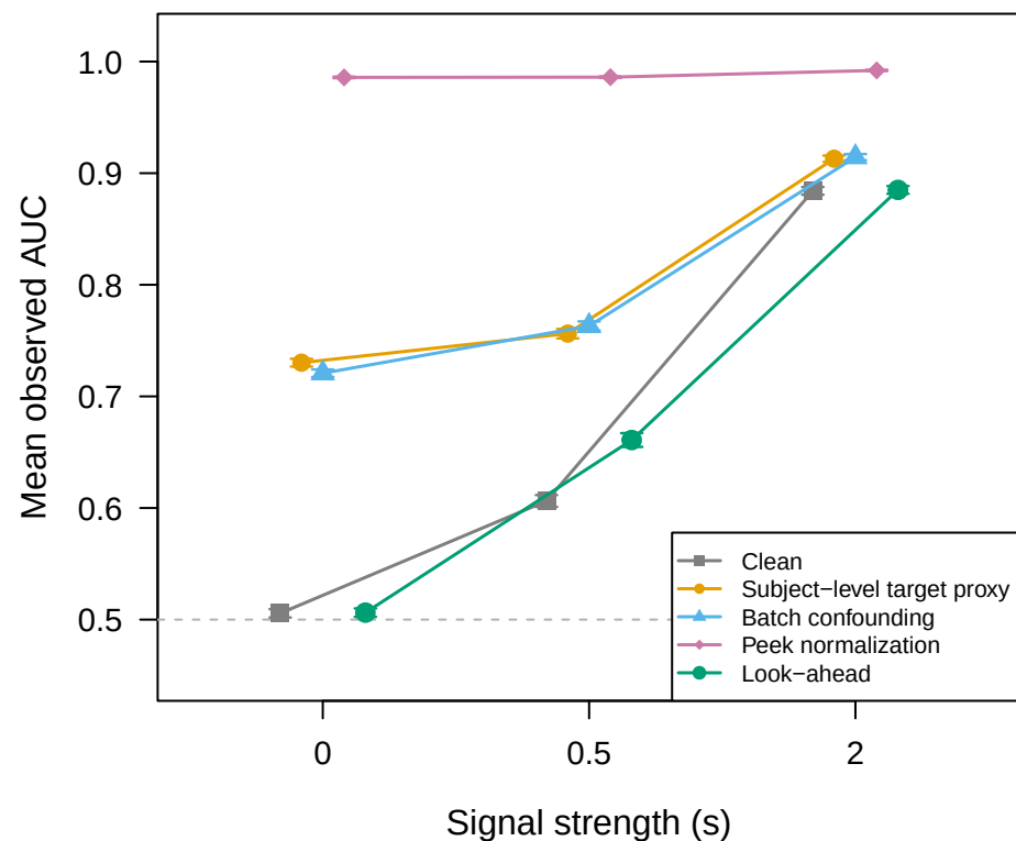
(d) AUC inflation vs clean baseline
