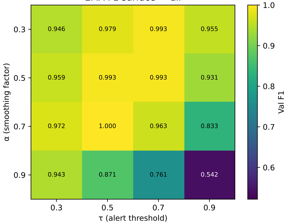
EMA F1 surface — all
