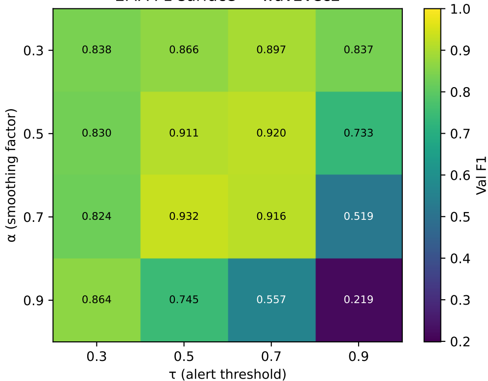
EMA F1 surface — wav2vec2
