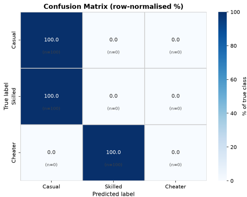
Figure 6: Confusion Matrix for Suspicion Scoring. Montre que l'algo de scoring n'arrive pas à différencier les profils de joueurs casual et expert. Il n'arrive pas également à différencier les profils de joueurs expert et cheater. Il est donc nécessaire de générer des profils plus réalistes pour que l'algo puisse apprendre à différencier les différents types de joueurs.
