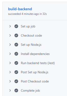
Figura 8.3: Pipeline de integración continua: Backend
