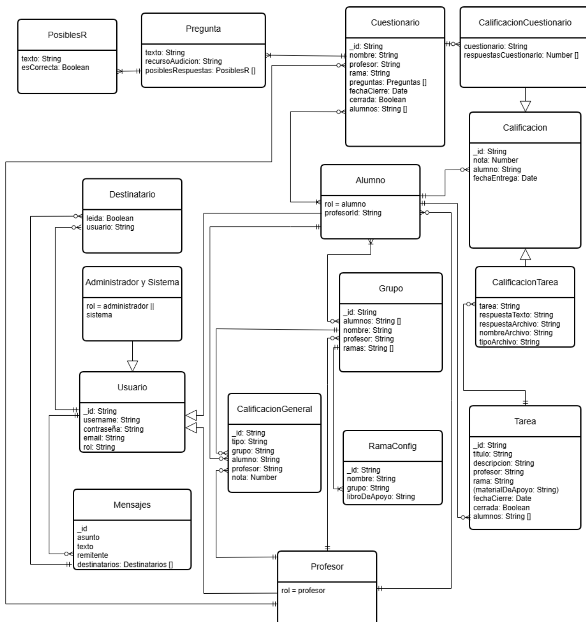
Figura 8.1: Modelo conceptual de datos del sistema
