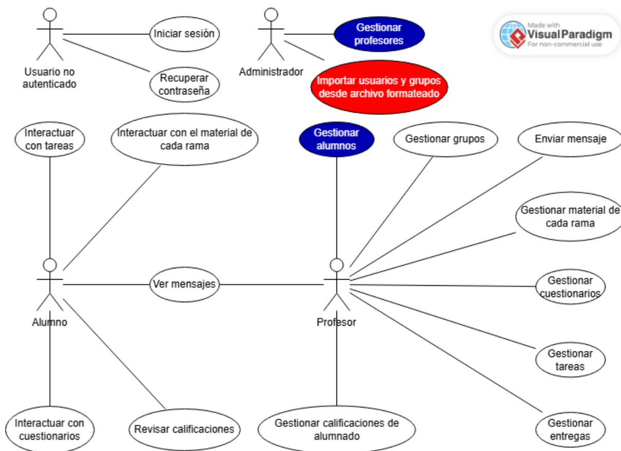
Figura 3.1: Diagrama UML de casos de uso del sistema extendido
