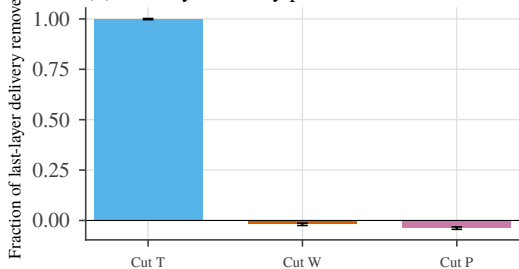
(d) Last-layer read by position
