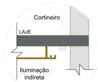
DETALHE CORTINEIRO + SANCA ILUMINADA
