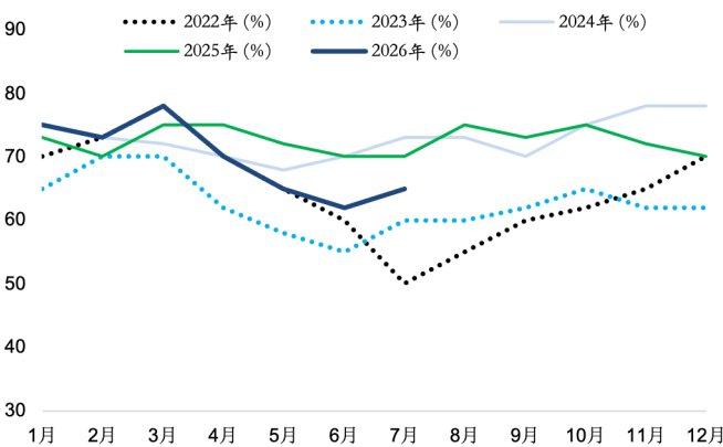
图 21: MEG 非煤制负荷
