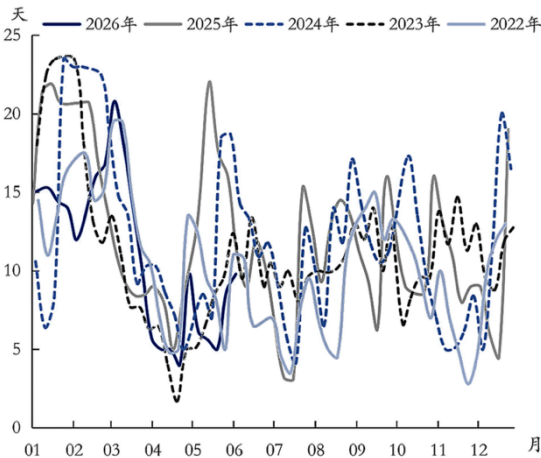
图 6: 织造聚酯原料库存天数
